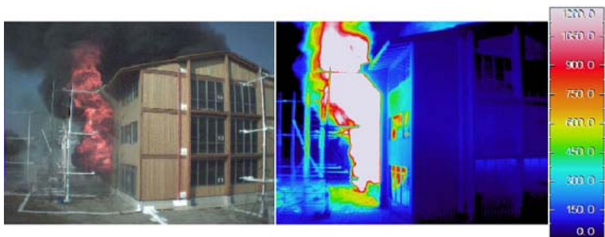
図 12 点火後 15 分の東側の熱映像と可視画像 (温度スケールの範囲は 0~1200℃)
