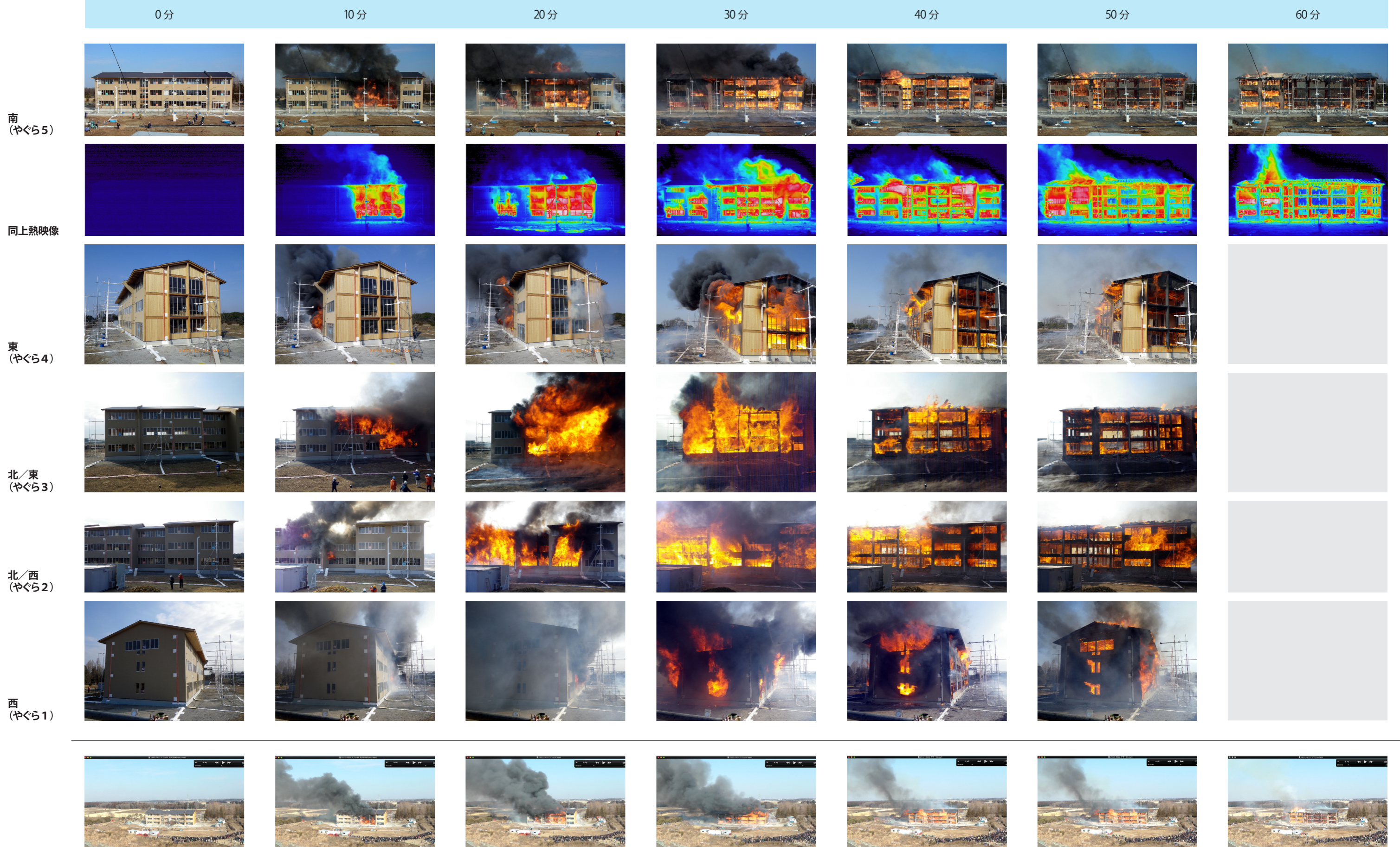
図16 点火後10分毎の映像（点火～60分）
