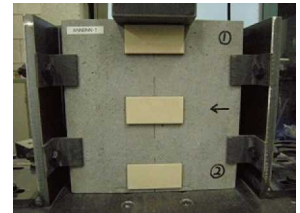
写真-2 せん断試験
