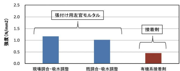
図-2 タイル直張りの直接引張り試験
