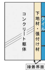
図-1 タイル外壁断面
