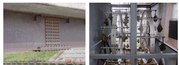
写真1 ボルトを使用した鋼橋の摩擦接合継手の例
