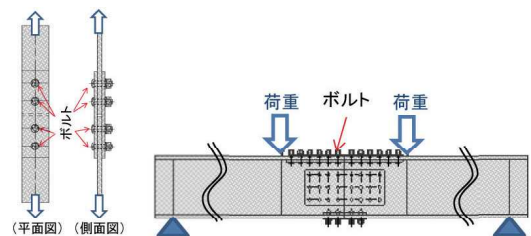
図1 標準すべり試験
