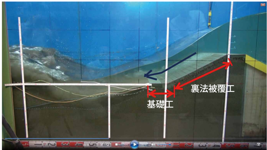
写真 裏法尻と裏法被覆工を工夫した構造の実験例
