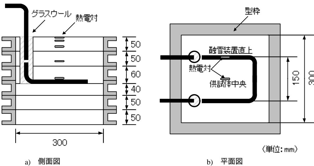
図-4 熱電対設置位置（温水パイプ方式，埋設深さ160mm）
