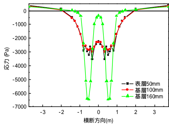
b) 電熱線
