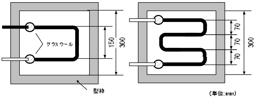
図-2 室内試験用供試体（側面図）
