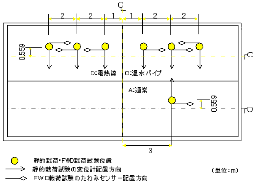
図-20 静的荷重・FWD荷重試験位置図
