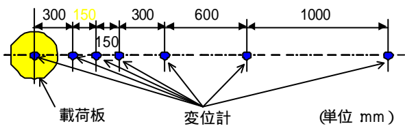
図-21 静的荷重試験とFWD荷重試験での変位測定位置
