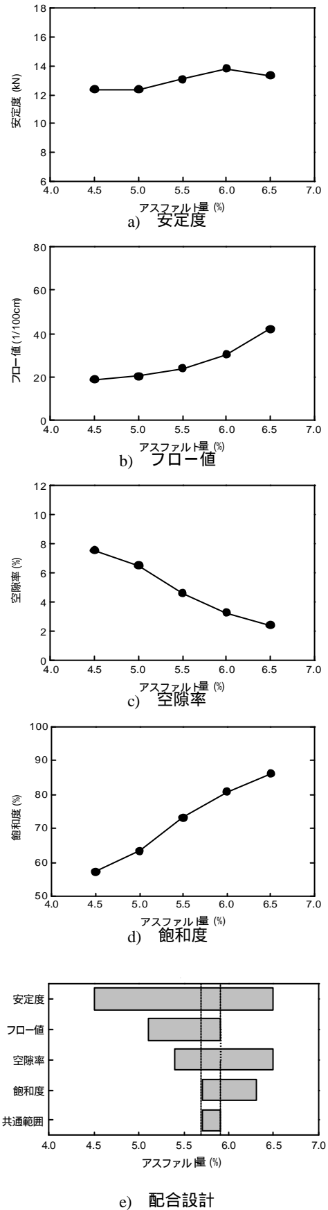
図-7 マーシャル安定度試験の結果
