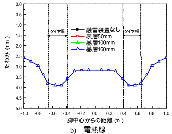
図-41 車輪中心位置における横断方向たわみ分布
