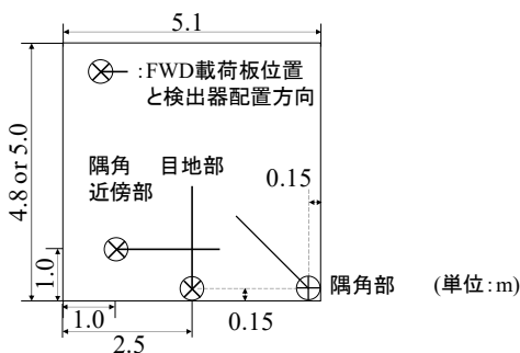
図-3.21 載荷板設置位置とたわみ検出器の配置方向
