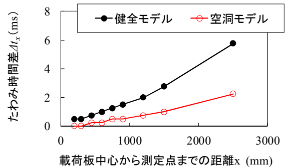
図-3.10 たわみ時間差の解析結果
