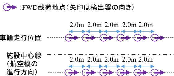
図-8.2 地震後の空港舗装における FWD の載荷地点の例
