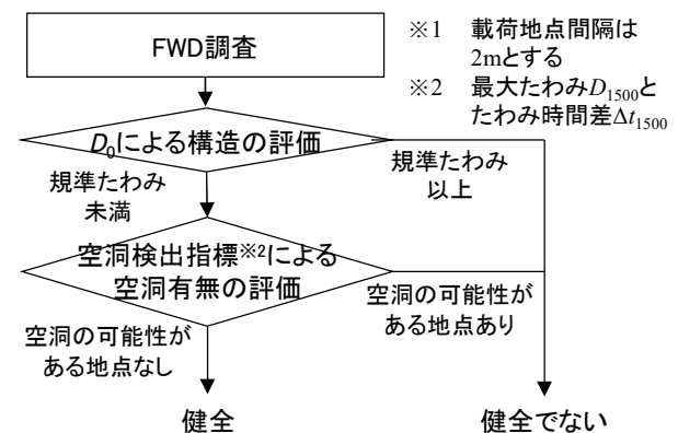
図-8.4 空洞が生じた空港アスファルト舗装の FWD による評価フロー
