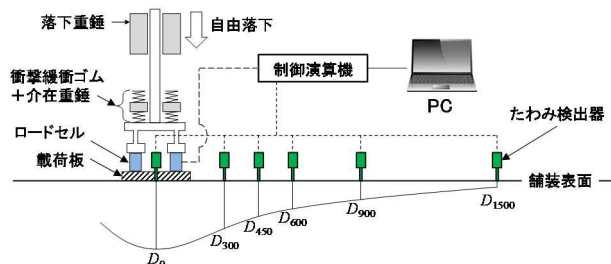
図-2.1 FWDの荷重機構の概念図
