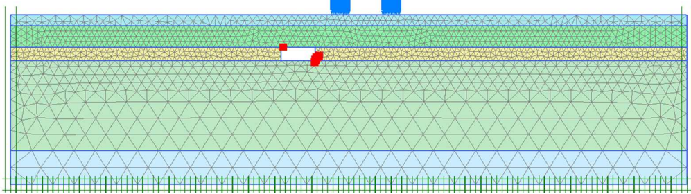
a) 空洞中心と左荷重中心の距離が 1.5m
