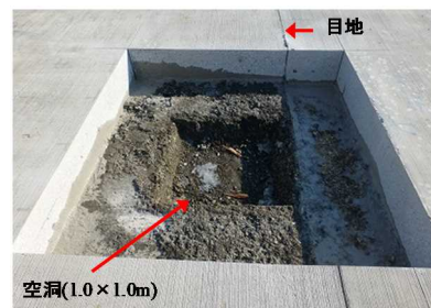
写真-4.1 空洞の生成状況(目地部 1.0x1.0m の空洞)
