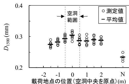
図-6.14 各載荷地点における最大たわみ D_{1500}
