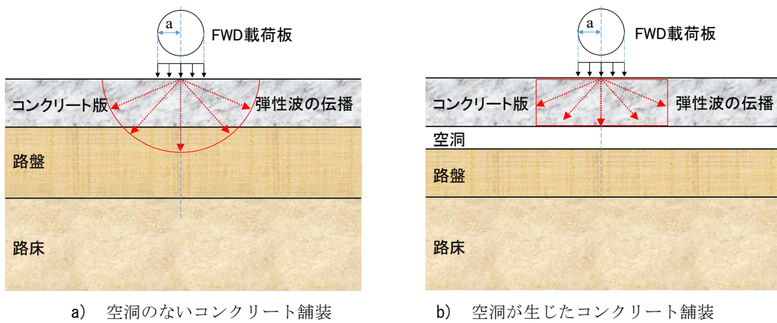
図-3.14 コンクリート舗装における弾性波の伝播イメージ
