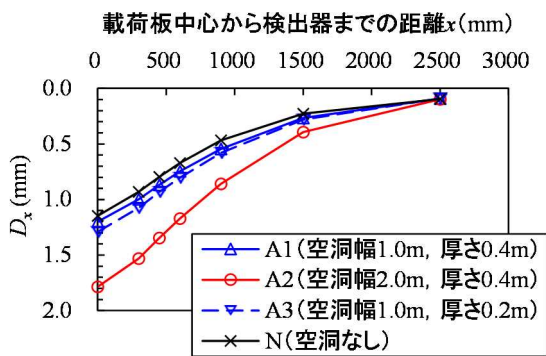
図-6.4 最大たわみ D_x
