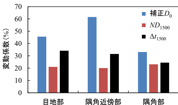
図-3.27 非空洞版群の各載荷位置での各指標の変動係数
