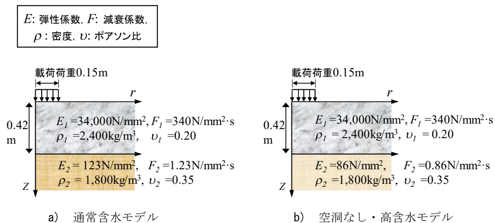
図-3.36 解析モデル
