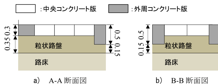
図-4.2 試験舗装の断面図
