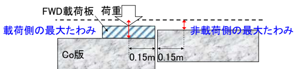
図-4.18 コンクリート版の目地部における FWD 調査イメージ
