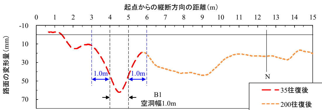
図-7.3 35往復後のBNレーンの変形量
