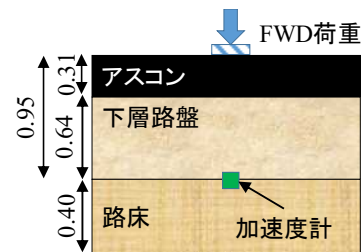
図-3.32 加速度計の設置位置
