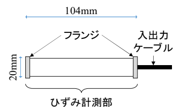
図-4.4 ひずみ計の模式図
