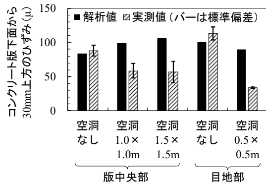
図-4.21 コンクリート版に生じたひずみの解析値と実測値
