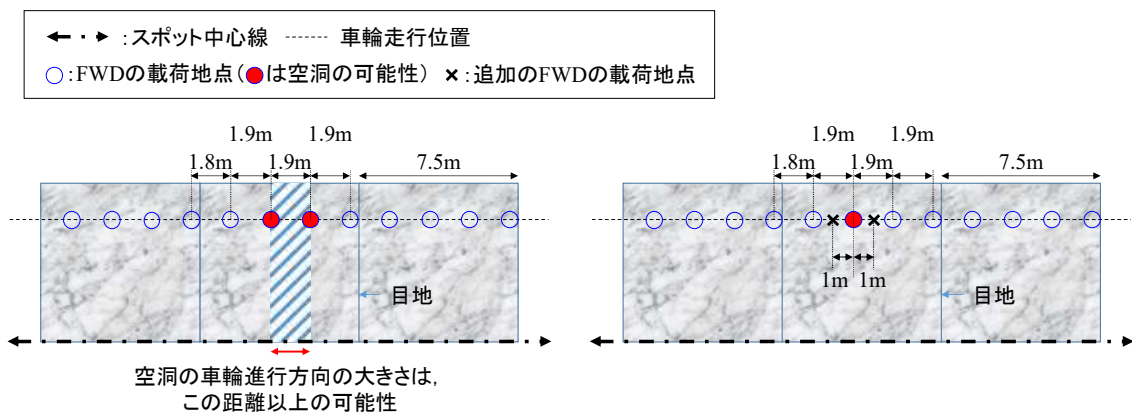
図-4.37 FWDによる空洞範囲の推定イメージ
