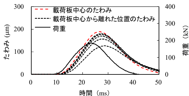
図-2.2 FWDで得られるデータの例
