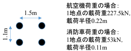
図-7.17 GAMES における荷重条件 (上から見た図)
