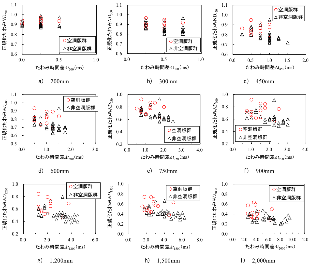
図-3.24 目地部の正規化たわみとたわみ時間差の関係
