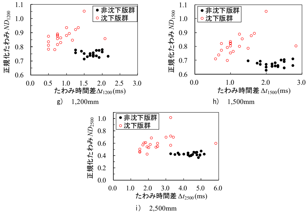
図-3.7 正規化たわみとたわみ時間差の関係
