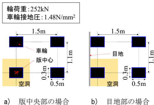
図-4.18 コンクリート版の目地部における FWD 調査イメージ
