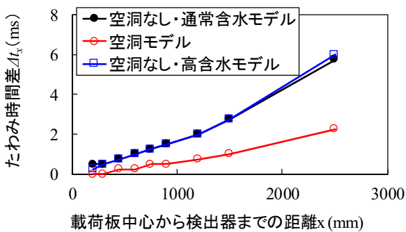
図-3.38 たわみ時間差の解析結果
