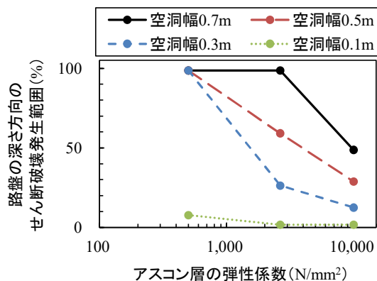
図-7.28 深さ方向のせん断破壊発生範囲率に対するアスコン層の空洞幅の影響
