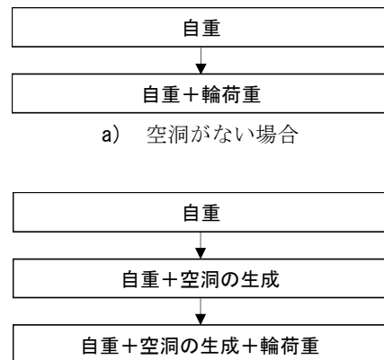
b) 空洞がある場合
