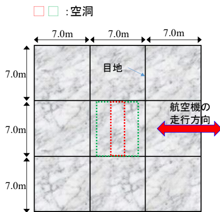
a) 空洞の位置が版中央部の場合
