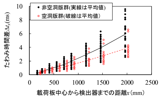
図-3.23 目地部のたわみ時間差
