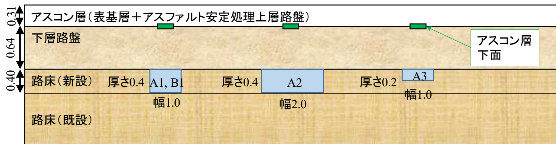
図-7.1 試験舗装の平面図と断面図
