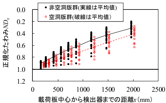
図-3.22 目地部の正規化たわみ
