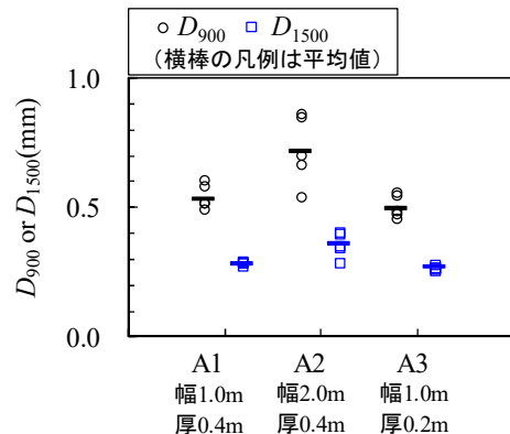
図-6.6 最大たわみ D_{900} および D_{1500}
