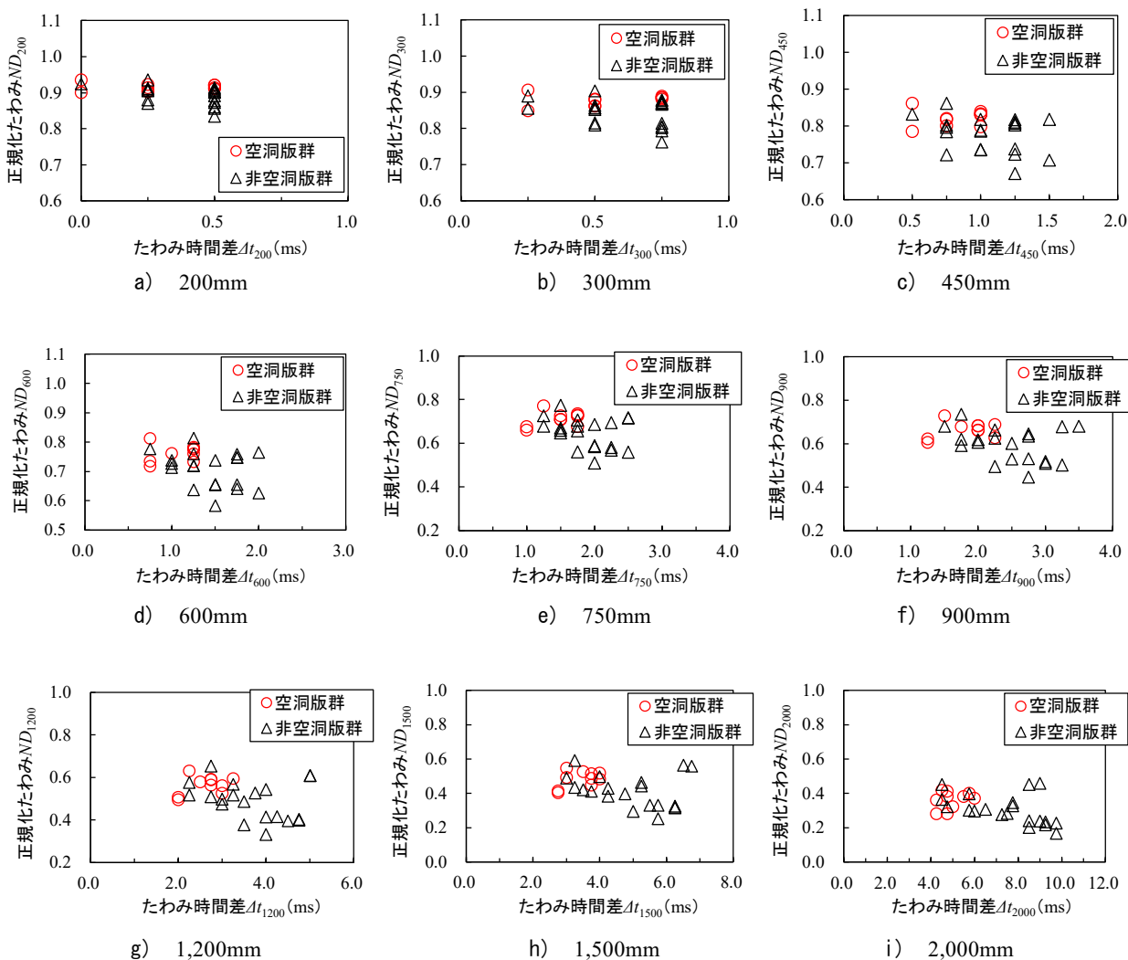
図-3.26 隅角部の正規化たわみとたわみ時間差の関係
