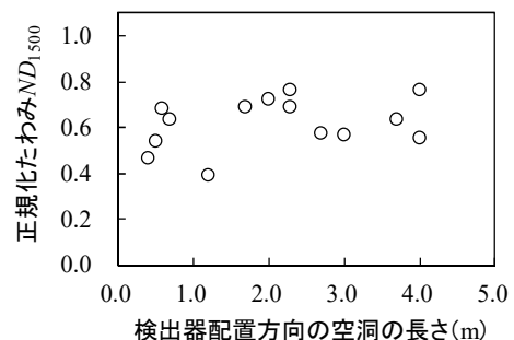
図-3.28 検出器配置方向の空洞の長さ( m) と正規化たわみ ND_{1500} の関係
