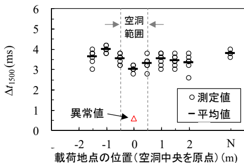
図-6.15 各載荷地点におけるたわみ時間差 \Delta t_{1500}
