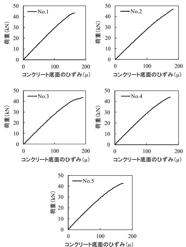
図-4.24 曲げ試験における荷重とコンクリート底面のひずみの関係
