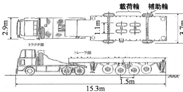
図-4.6 荷重車の全体図
