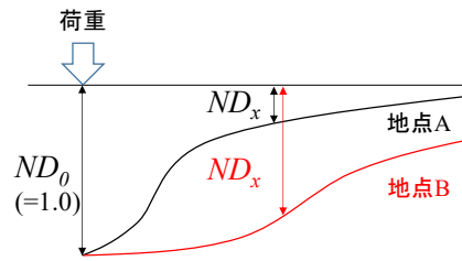
b) 正規化たわみ ND_0 ( x = 0 \sim 200 mm)
