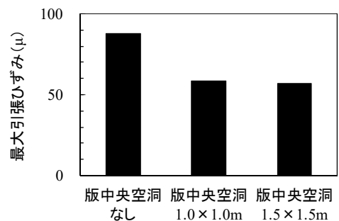
図-4.10 98~100 往復時の版中央部下面の最大引張ひずみ
