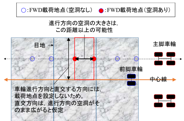
図-4.27 FWDで推定される空洞の形状イメージ
