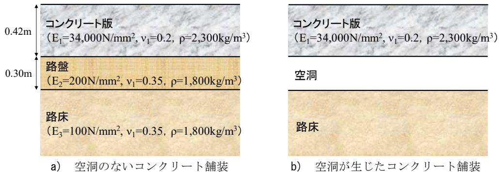
図-3.17 弾性波の伝播速度の算出のための舗装モデル
