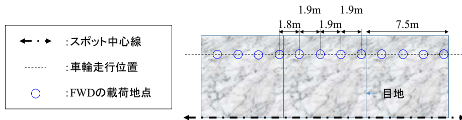
図-4.36 地震後の空港コンクリート舗装におけるFWDの荷地点
