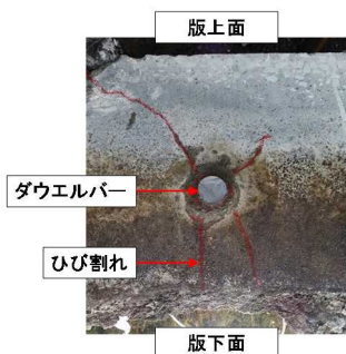
写真-4.4 1.0×1.0mの空洞上のコンクリート版目地の断面
