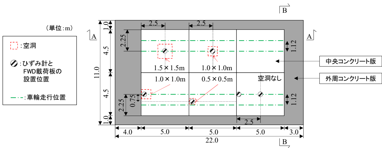
図-4.1 試験舗装の平面図
