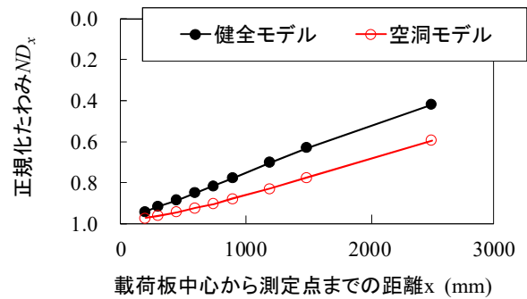
図-3.9 正規化たわみの解析結果
