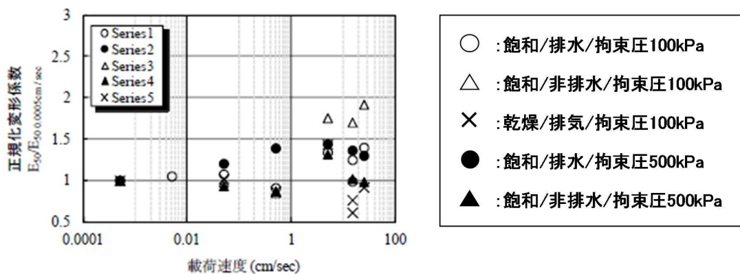
図-3.31 荷速度と正規化変形係数の関係 19) (凡例の補足を加筆)
