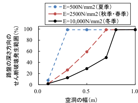
図-7.29 深さ方向のせん断破壊発生範囲率に対するアスコン層の弾性係数の影響
