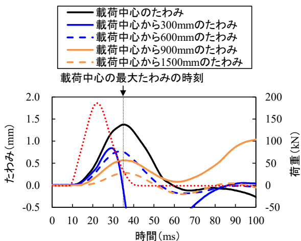
図-6.16 各載荷地点におけるたわみ時間差 \Delta t_{1500}
