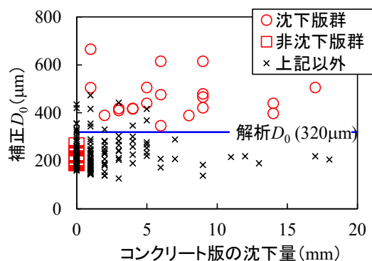
図-3.2 沈下量と補正 D_0 の関係
