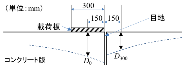
図-2.4 目地部での FWD の載荷板設置位置
