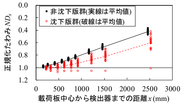
図-3.5 正規化たわみ
