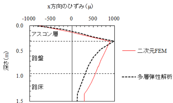
a) 左側荷重の中心における \epsilon_x の深さ方向の分布
