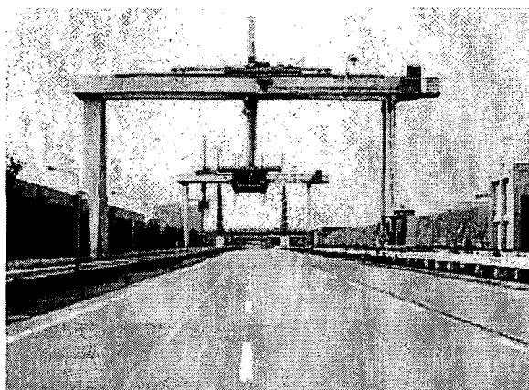
標識屋外実験施設外観
