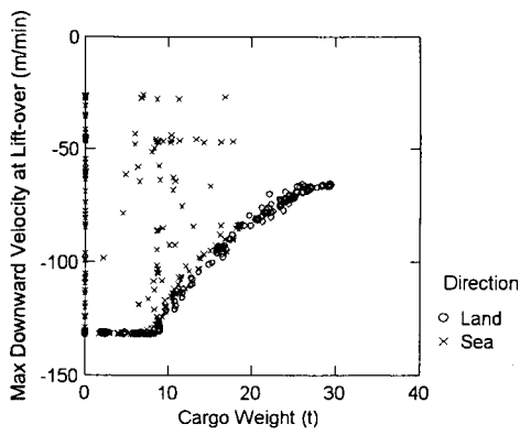
図- 52 吊荷重と最大巻下速度 (PP 船)
