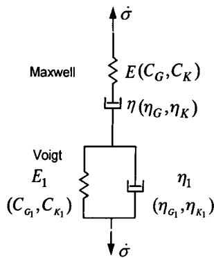
図-16 Burger モデル
