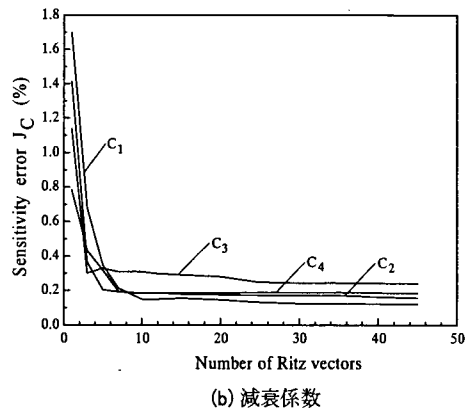
図-4 Ritzベクトル数と弾性係数・減衰係数
