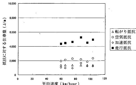
図-56 走行抵抗に対する仕事量の内訳 (高速道路走行・14.0t)
