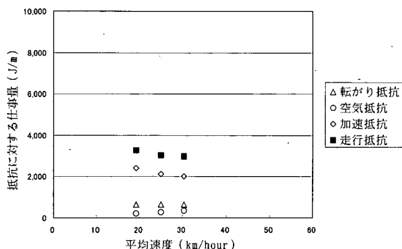
図-54 走行抵抗に対する仕事量の内訳 (一般道路走行・6.6t)
