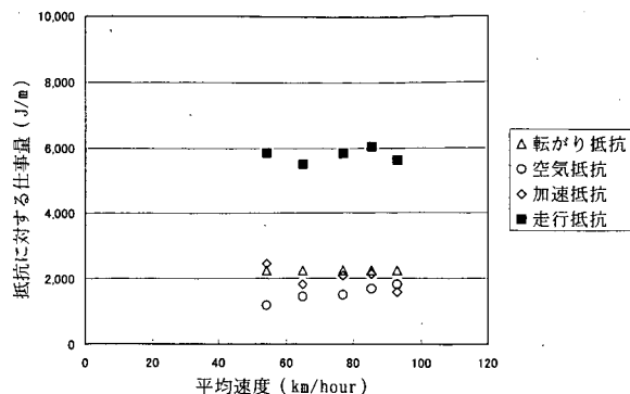
図-55 走行抵抗に対する仕事量の内訳 (高速道路走行・22.8t)
