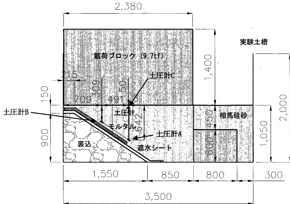
図-G.2 土圧計設置箇所
