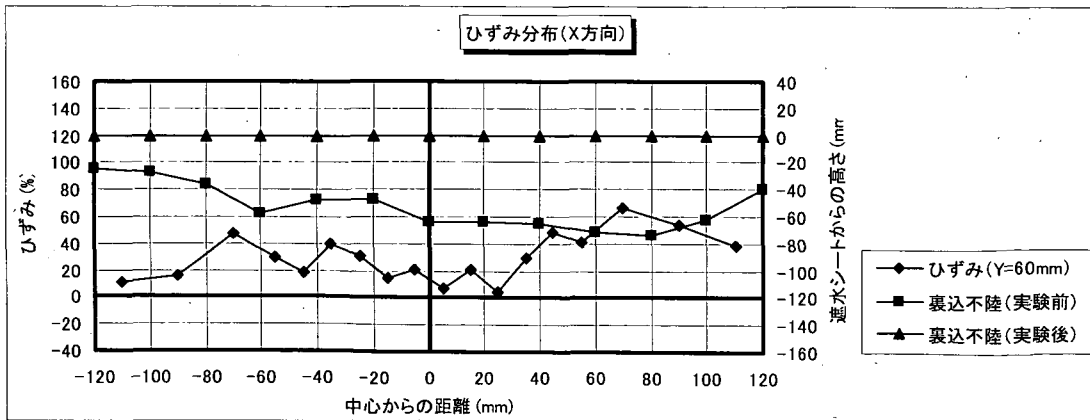
図-F.12_4 遮水シート線ひずみ分布 (X方向分布: 丸形・配列①; ケース4-8)
