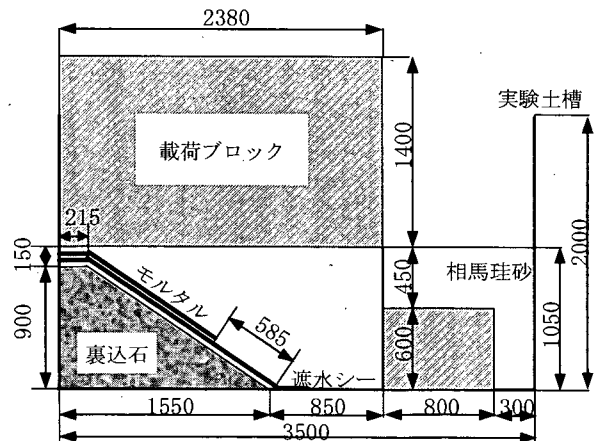
(b) 断面図
