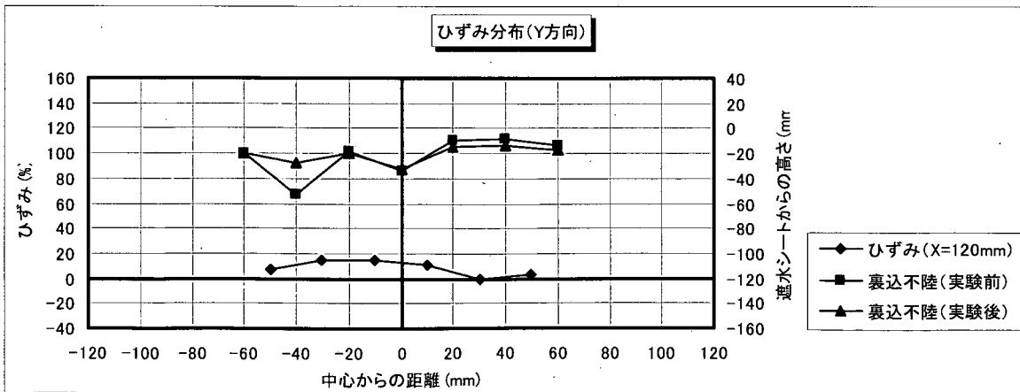
図-F.9_5 遮水シート線ひずみ分布 (Y方向分布: 角形・配列②; ケース4-6)
