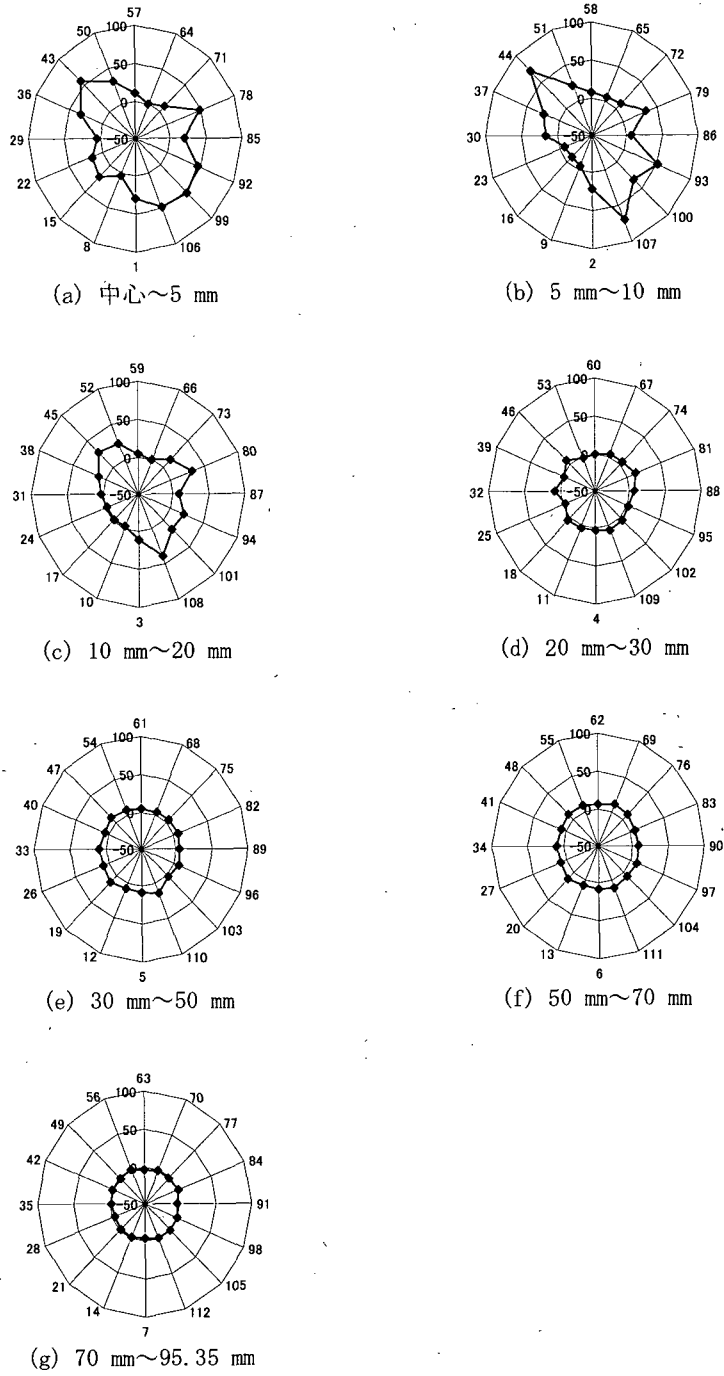
図-E.17 遮水シート線ひずみ分布 (円周方向ひずみ : 円周方向分布 : 丸形② ; ケース3-13)
