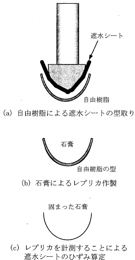
図-3.2 遮水シートのひずみ計測のための型取り
