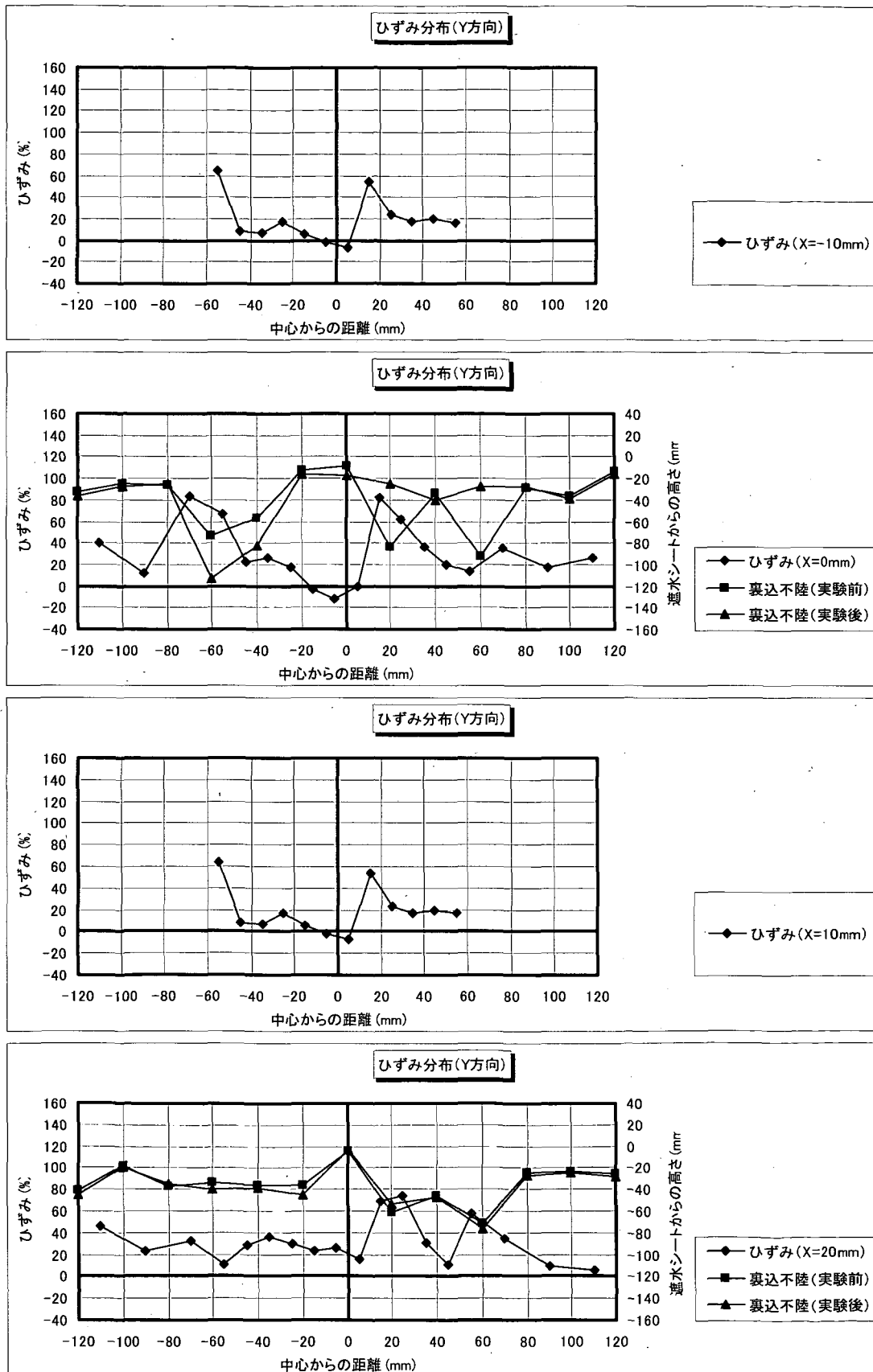
図-F.9_3 遮水シート線ひずみ分布(Y方向分布:角形・配列②; ケース4-6)
