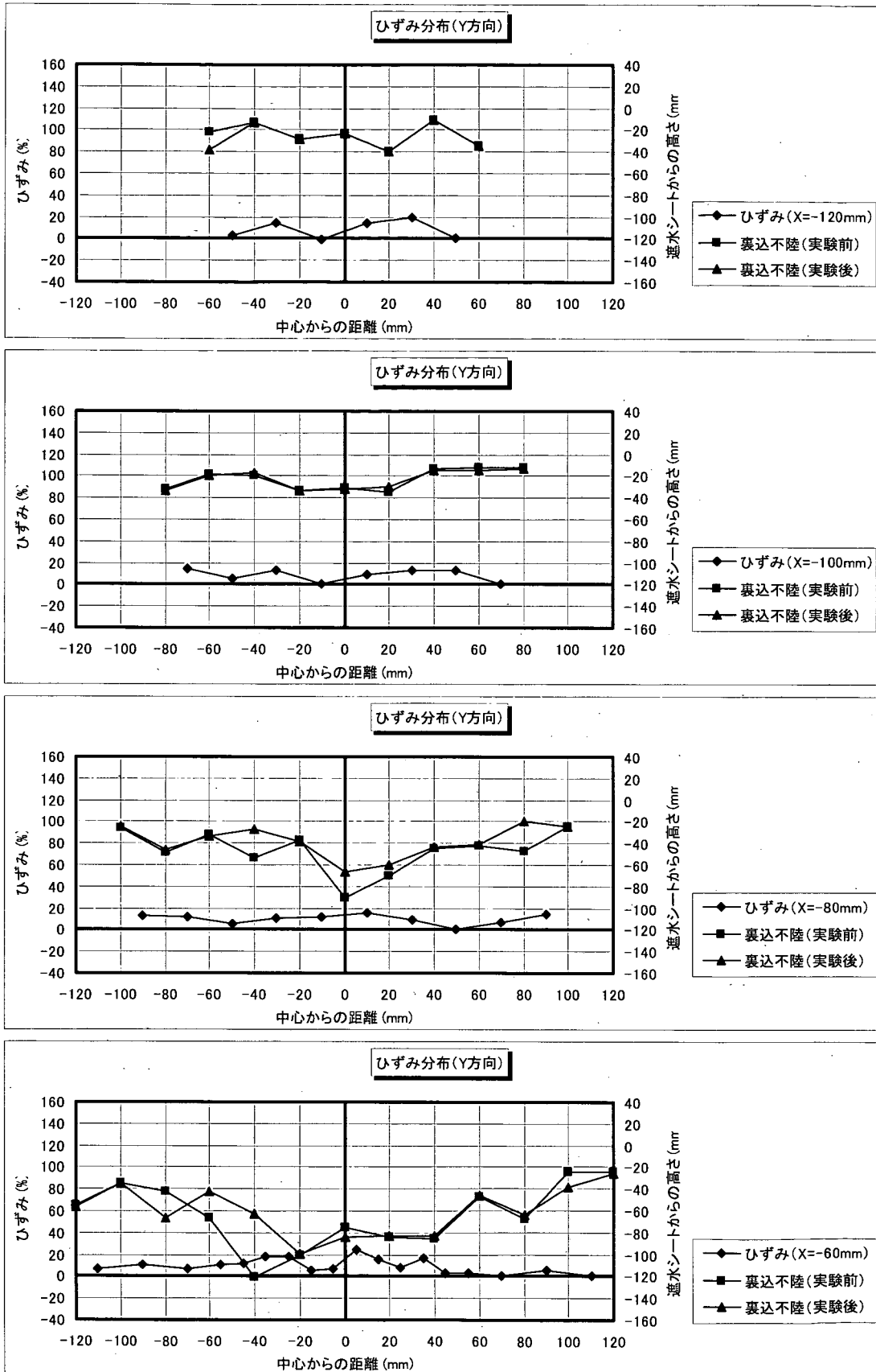
図-F.5_1 遮水シート線ひずみ分布 (Y方向分布: 角形・配列①; ケース4-3)
