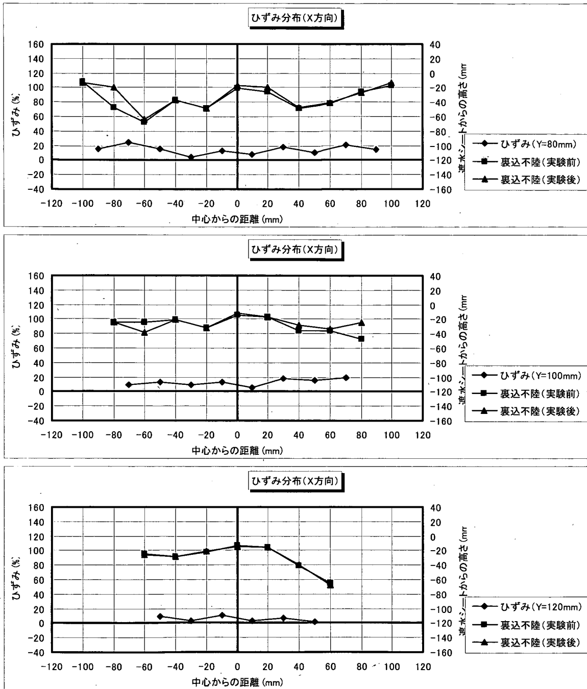
図-F.4_5 遮水シート線ひずみ分布 (X方向分布: 角形・配列①; ケース4-3)
