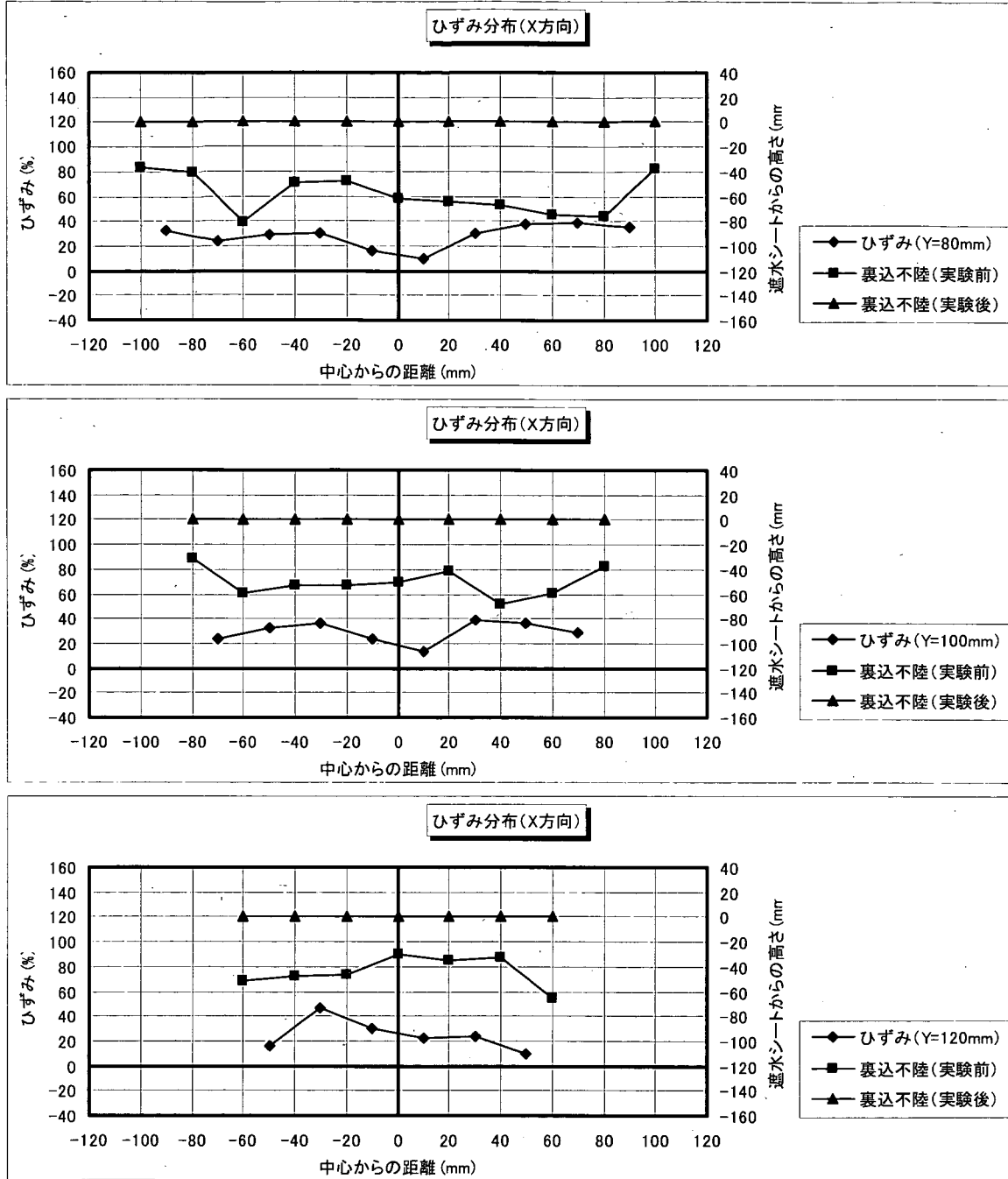
図-F.12_5 遮水シート線ひずみ分布 (X方向分布: 丸形・配列①; ケース4-8)
