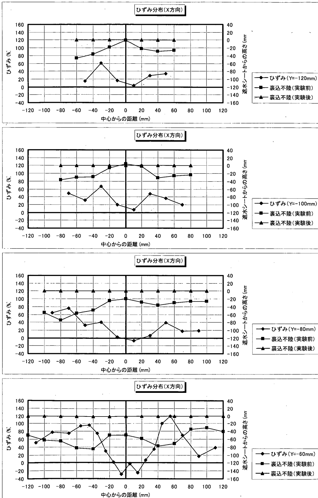
図-F.12.1 遮水シート線ひずみ分布 (X方向分布: 丸形・配列①; ケース4-8)
