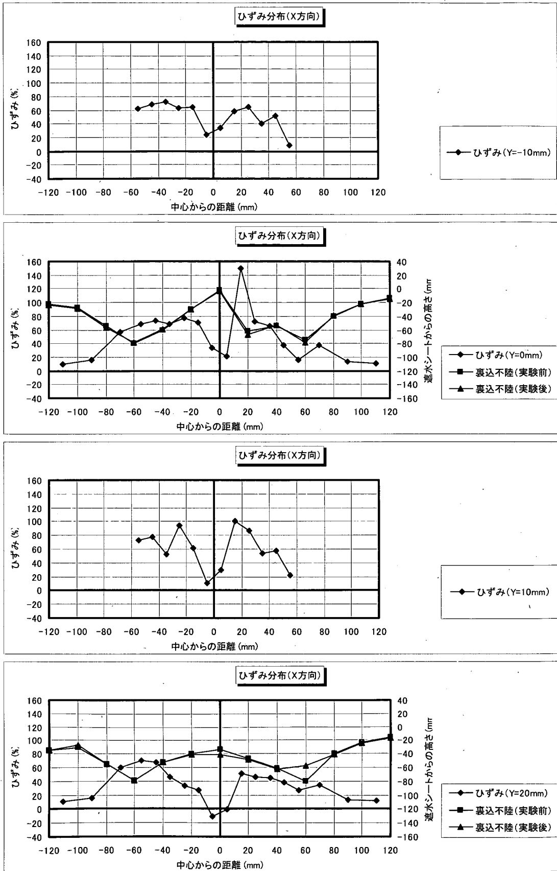
図-F.6_3 遮水シート線ひずみ分布 (X方向分布: 角形・配列①; ケース4-5)
