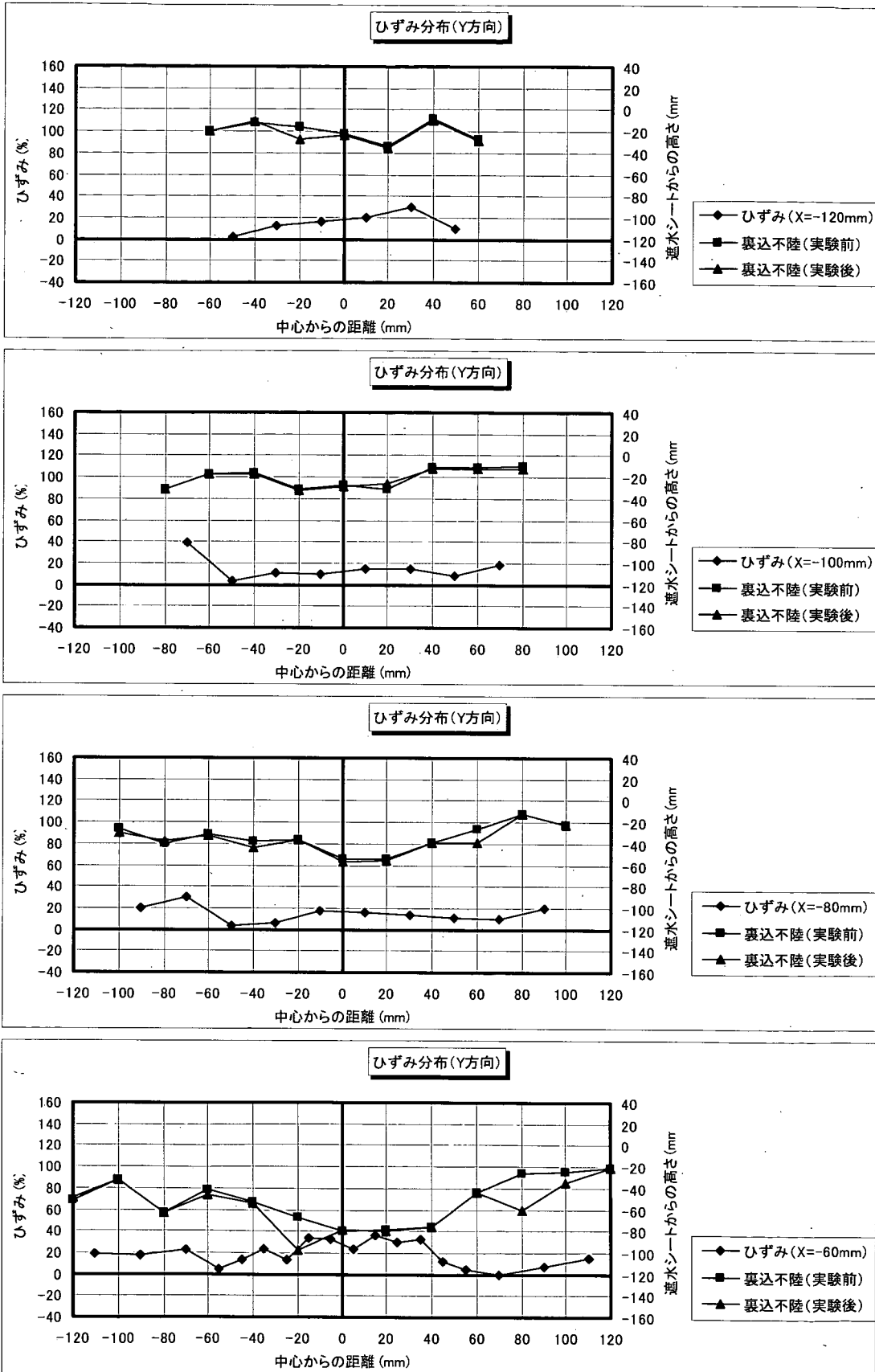
図-F.7_1 遮水シート線ひずみ分布 (Y方向分布: 角形・配列①; ケース4-5)
