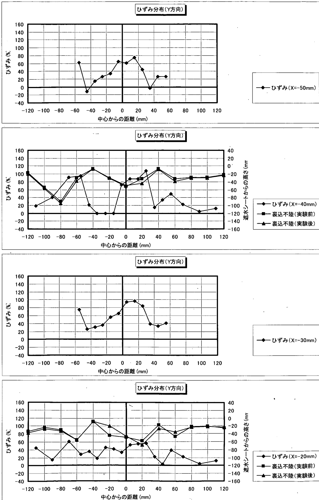
図-F.9_2 遮水シート線ひずみ分布 (Y方向分布: 角形・配列②; ケース4-6)
