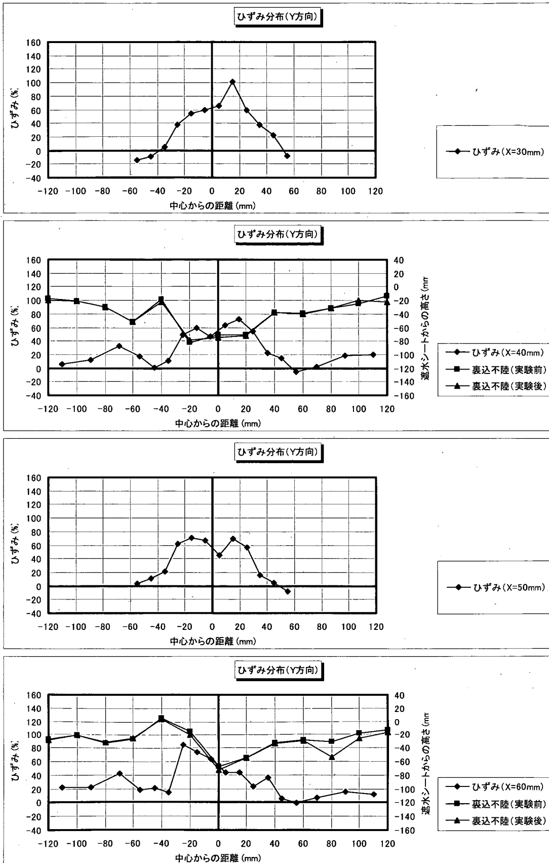
図-F.11_4 遮水シート線ひずみ分布 (Y方向分布: 角形・配列③; ケース4-7)
