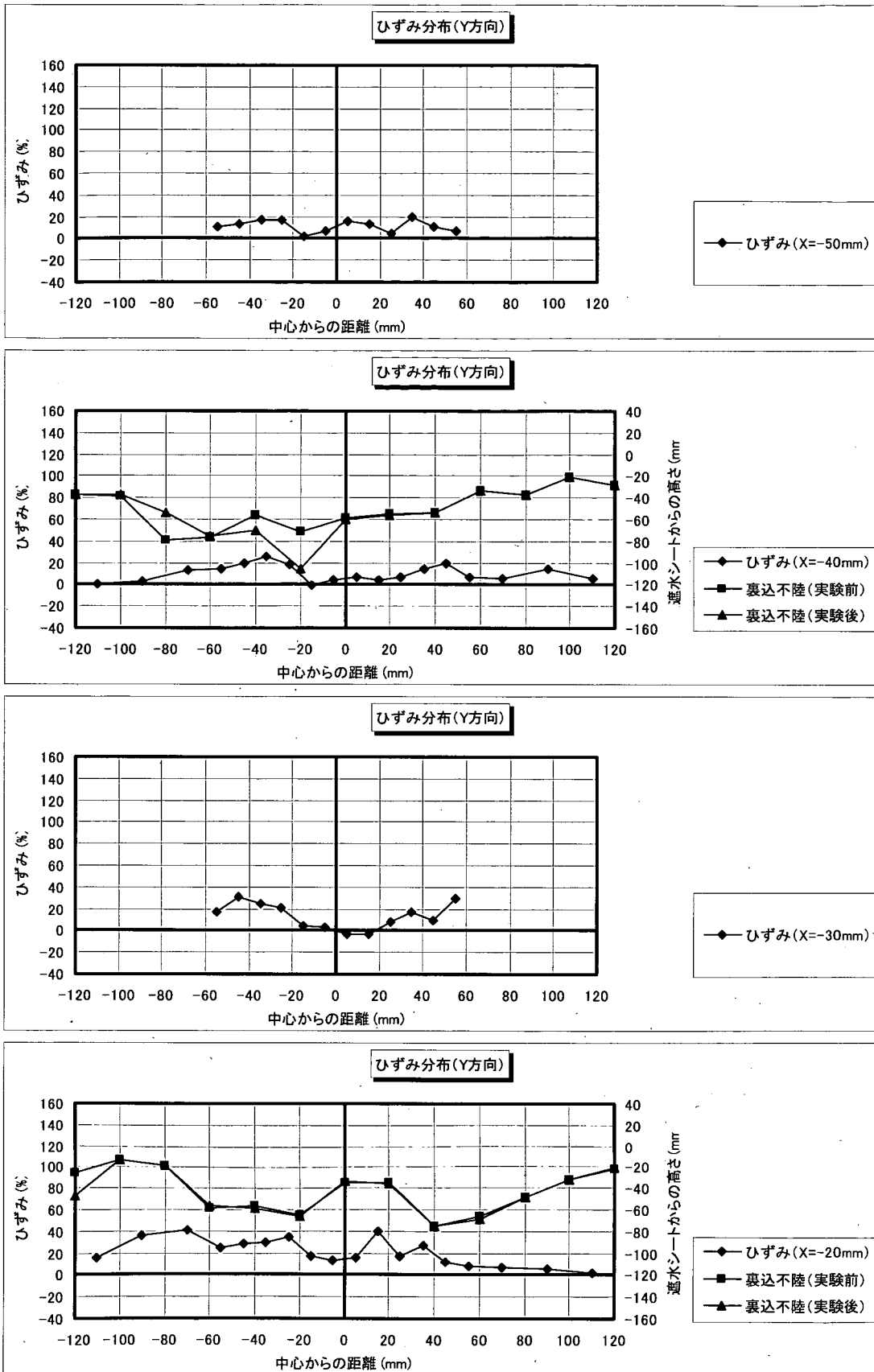
図-F.5_2 遮水シート線ひずみ分布 (Y方向分布: 角形・配列①; ケース4-3)
