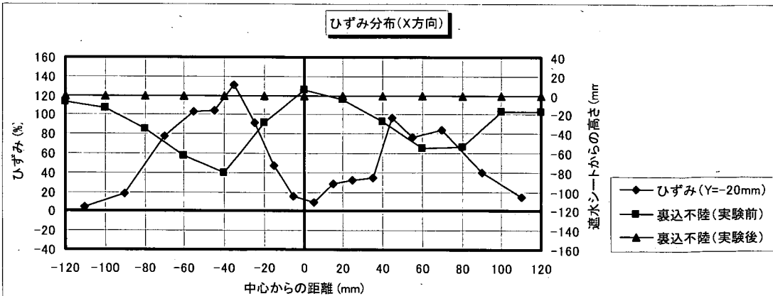
図-F.12_2 遮水シート線ひずみ分布 (X方向分布：丸形・配列①；ケース4-8)
