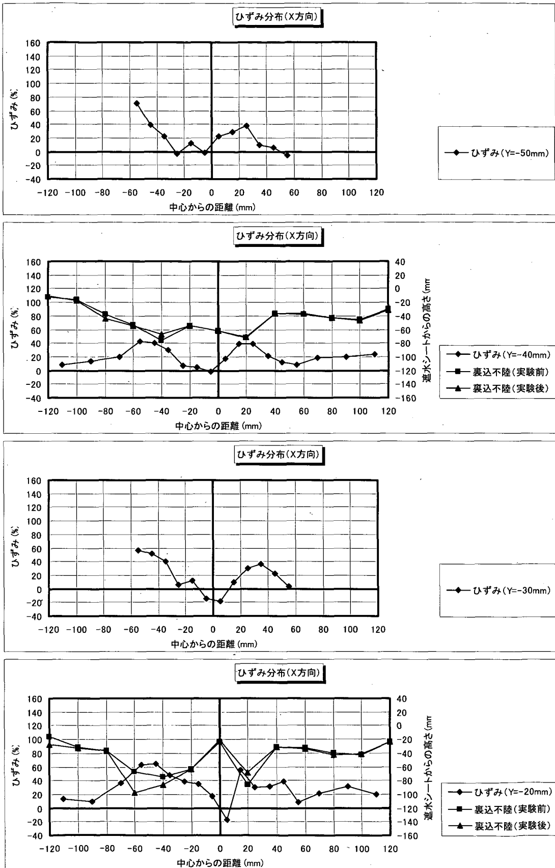
図-F.6.2 遮水シート線ひずみ分布 (X方向分布: 角形・配列①; ケース4-5)
