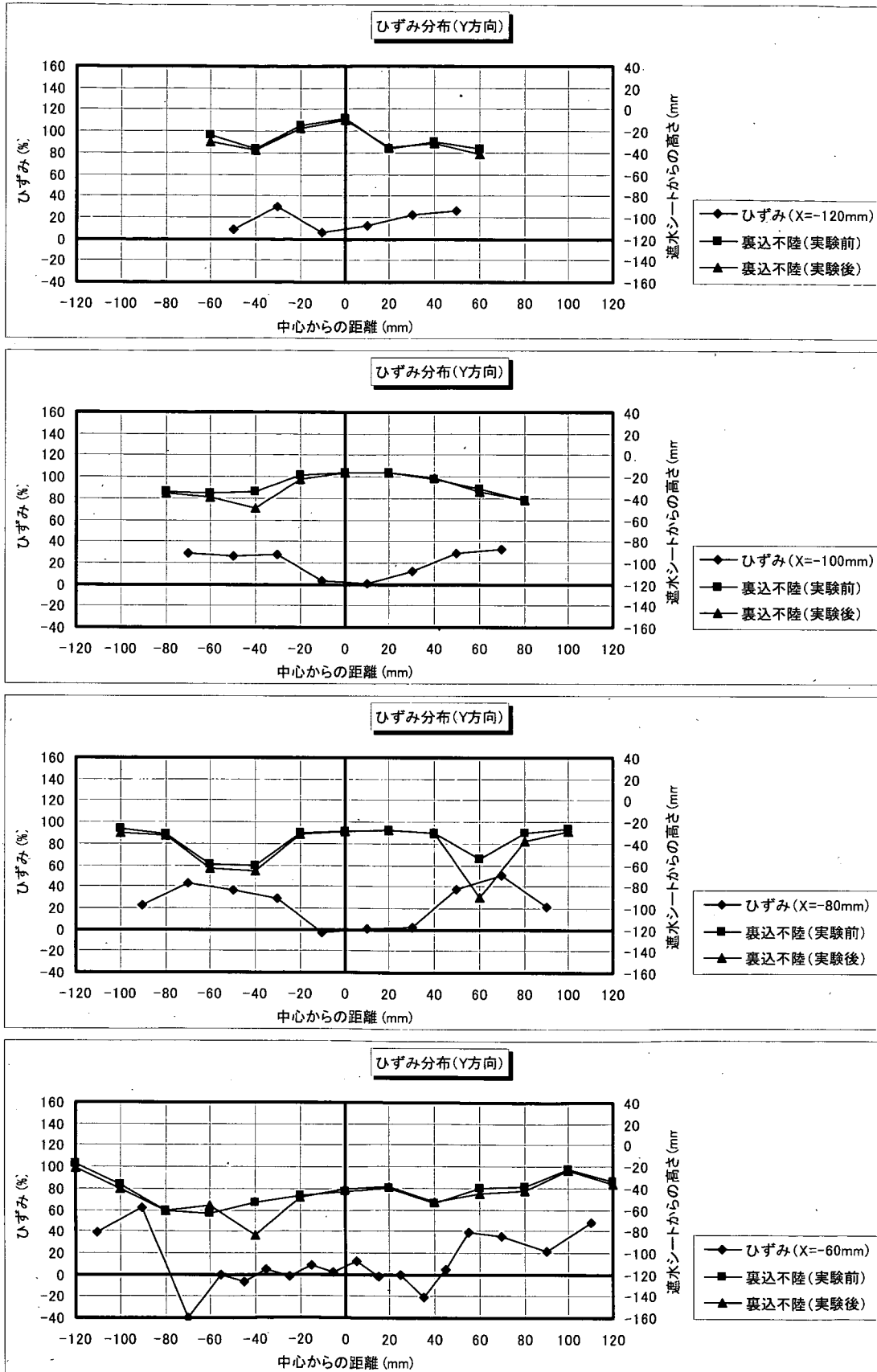
図-F.9_1 防水シート線ひずみ分布 (Y方向分布: 角形・配列②; ケース4-6)
