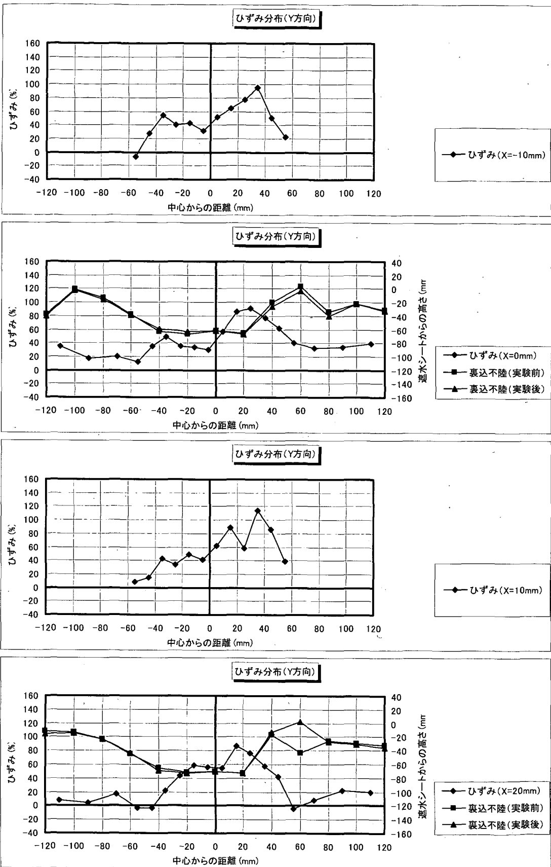
図-F.11_3 遮水シート線ひずみ分布 (Y方向分布: 角形・配列③; ケース4-7)
