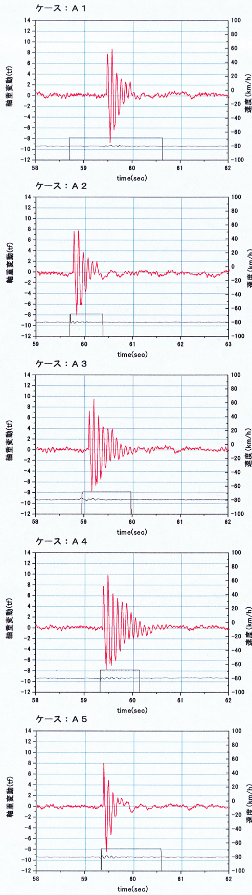
図-2.4.19 (b) 単独段差試験軸重波形 (段差高さ 30mm [斜路あり] 速度 80km/h 1 回目走行)
