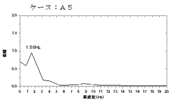
図-2.5.5(b) 軸重変動波形の周波数特性 (段差高さ 100mm 速度 5km/h 1回目走行)
