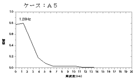
図-2.5.6(b) 軸重変動波形の周波数特性 (段差高さ 60mm 速度 10km/h 1 回目走行)
