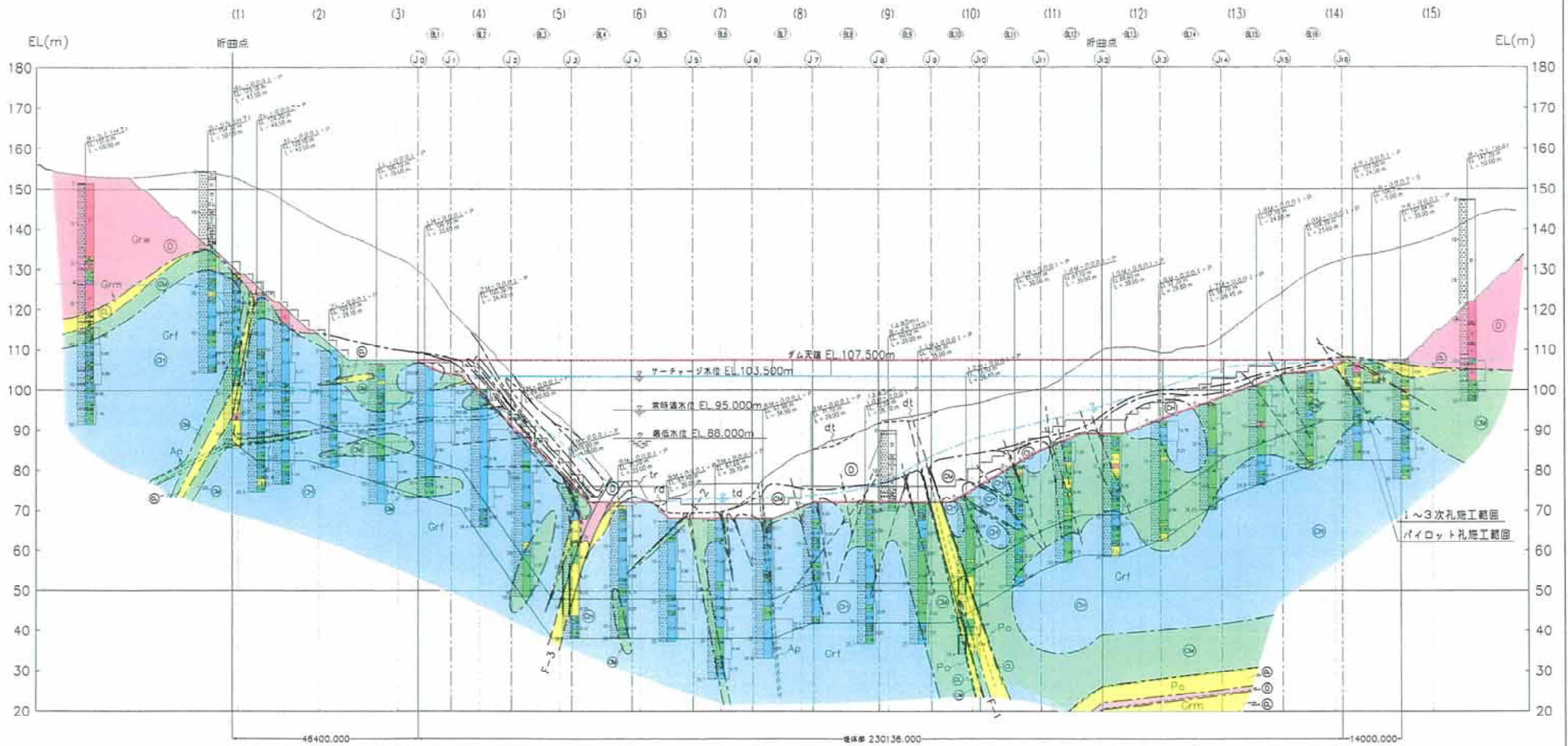
ダム軸（止水ライン）断面図
