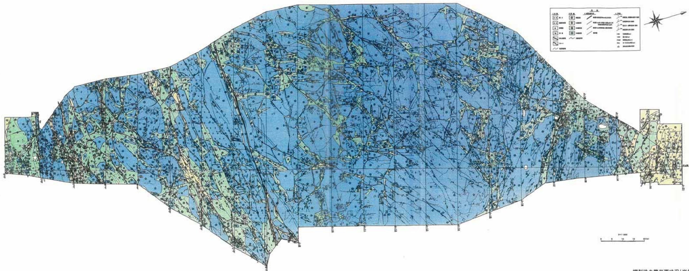
掘削後の着岩面状況(岩級)
