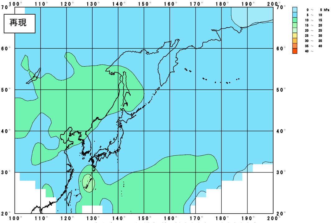
図-51 低気圧の中心気圧の標準偏差(上:実測, 下:再現)
