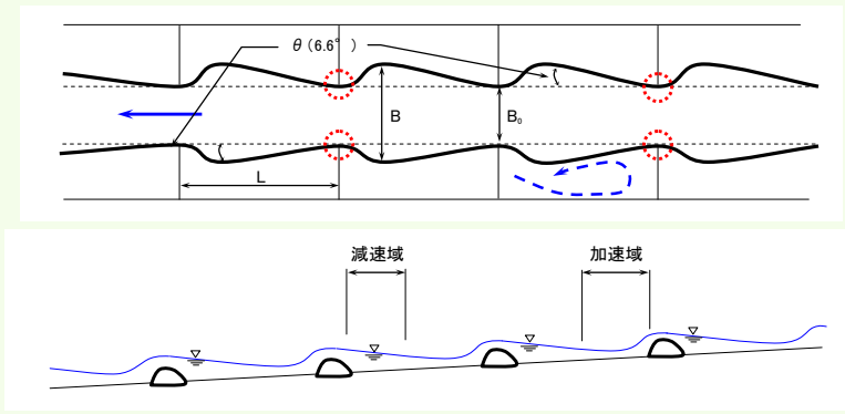
図 5-35 水制工の配置間隔と水理特性(長野県建設部砂防課, 2009)
