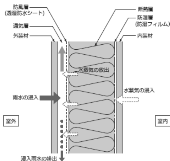
図1 建物外皮の基本構成(外壁縦断面)
