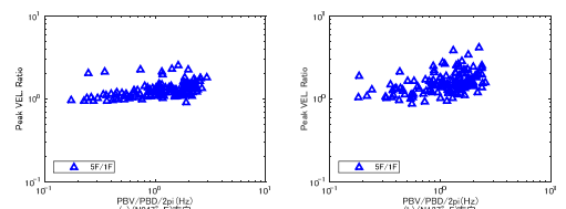
図 4.4 等価卓越振動数 (fv) と最大速度比 (SF/1F) の関係
