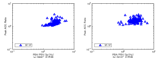
図 4.3 等価卓越振動数 (fa) と最大加速度比 (SF/1F) の関係
