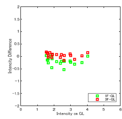
図 3.6 GL の最大震度と 1F/GL 及び 3F/GL の計測震度差の関係
