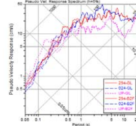
図 7.4 地表 (GL) と B2 階 (B2F) の記録の擬似速度応答スペクトル (h=5%)
