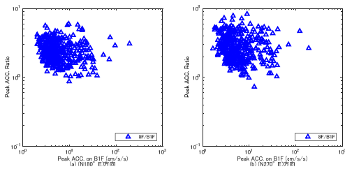
図 3.10 BIF の最大加速度と 8F/BIF の最大加速度比の関係
