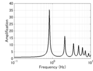
図 1.1 工業的基礎に対する地盤の伝達関数
