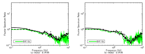
図 6.11 311地震と震度2の地震の比較(B1F/G1) ※実線: 本震後、破線: 本震前
