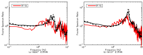
図 6.8 311 地震と震度 2 の地震の比較 (5F/GL) ※実線: 本震後、破線: 本震前
