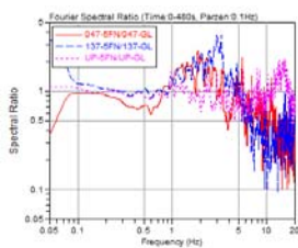
図 7.6 5 階 (O5F) の地表 (GL) に対するフーリエ振幅スペクトル比
