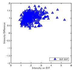
図 3.12 BIF の計測震度と 8F-BIF の計測震度差の関係
