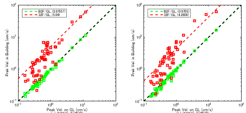
図 3.2 GL の最大速度と B2F 及び 32F の最大速度の関係
