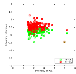
図 3.6 GL の最大震度と 1F/GL 及び 5F/GL の計測震度差の関係
