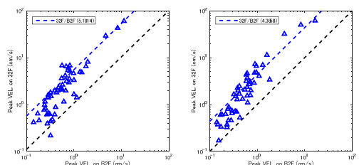
図 3.8 B2F の最大速度と 32F の最大速度の関係
