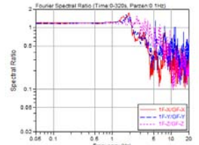
図 7.5 1階 (O1F) の地表 (GL) に対するフーリエ振幅スペクトル比
