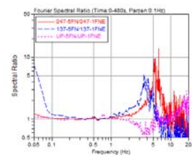
図 7.7 5 階 (O5F) の 1 階 (O1F) に対するフーリエ振幅スペクトル比
