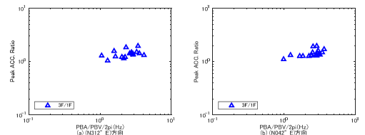
図 4.3 等価卓越振動数 (fa) と最大加速度比 (3F/1F) の関係
