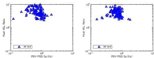
図 4.4 等価卓越振動数 (fV) と最大速度比 (RF/BIF) の関係
