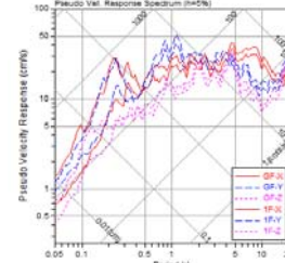
図 7.4 地表 (GL) と 1階 (O1F) の記録の擬似速度応答スペクトル (h=5%)
