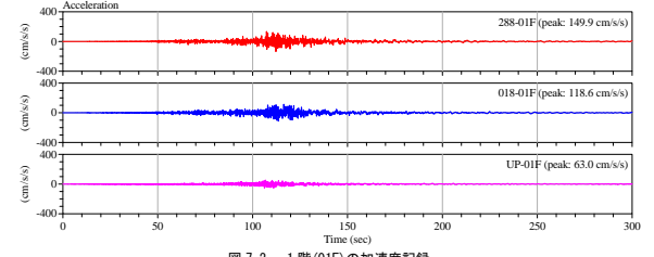
図 7.2 1階(01F)の加速度記録
