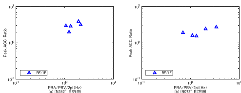
図 4.3 等価卓越振動数 (fa) と最大加速度比 (RF/IF) の関係
