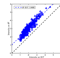
図 3.9 B1F の計測震度と 8F の計測震度の関係
