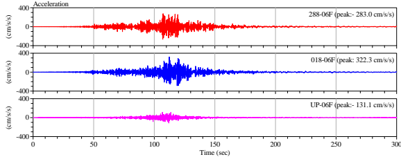
図 7.3 6階(06F)の加速度記録
