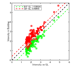
図 3.3 GL の計測震度と BIF 及び 32F の計測震度の関係
