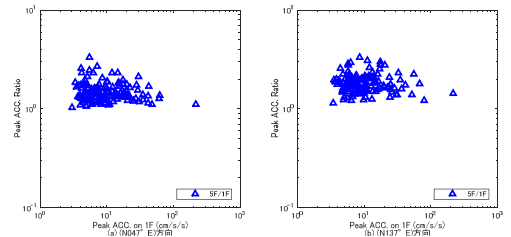
図 3.10 1F の最大加速度と SF/1F の最大加速度比の関係
