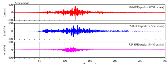
図 7.3 8 階 (8FE) の加速度記録
