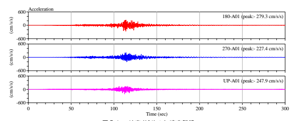
図 7.1 地表 (A01) の加速度記録
