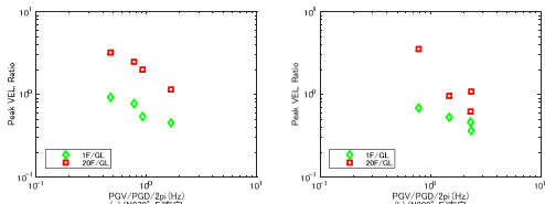
図 4.2 等価卓越振動数 (fV) と最大速度比 (20F/GL, 1F/GL) の関係
