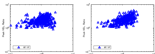
図 4.4 等価卓越振動数 (fv) と最大速度比 (6F/1F) の関係
