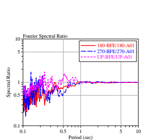
図 7.5 地下 1 階 (BFE) の地表 (A01) に対するフーリエ振幅スペクトル比
