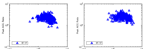
図 4.3 等価卓越振動数 (fa) と最大加速度比 (6F/1F) の関係
