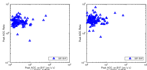
図 3.10 BIF の最大加速度と 32F/BIF の最大加速度比の関係
