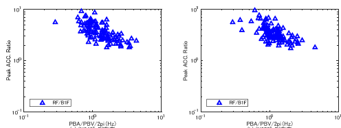
図 4.3 等価卓越振動数 (fA) と最大加速度比 (RF/BIF) の関係
