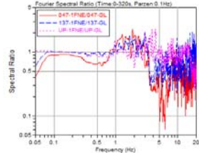
図 7.5 1 階 (O1F) の地表 (GL) に対するフーリエ振幅スペクトル比
