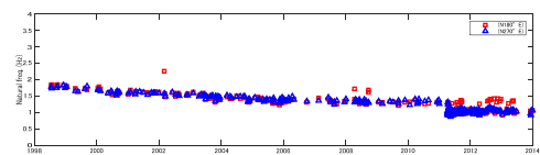
図 5.2 固有振動数 (8F/GL) の経年推移
