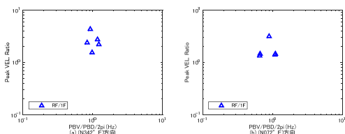
図 4.4 等価卓越振動数 (fv) と最大速度比 (RF/IF) の関係
