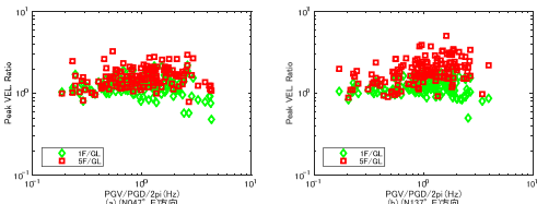
図 4.2 等価卓越振動数 (fv) と最大速度比 (SF/GL, 1F/GL) の関係
