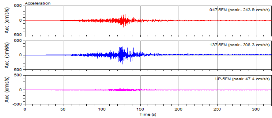
図 7.3 5 階 (O5F) の加速度記録
