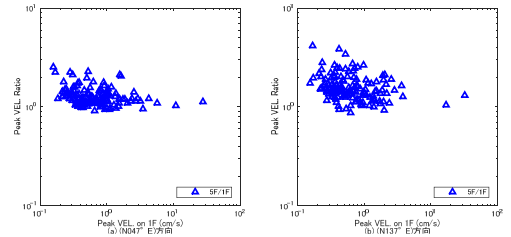
図 3.11 1F の最大速度と SF/1F の最大速度比の関係
