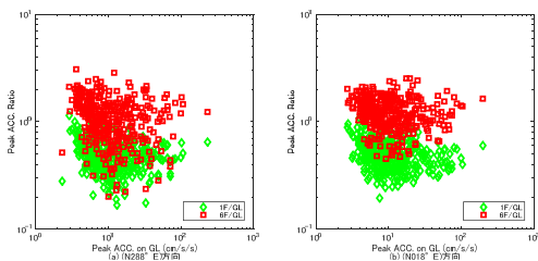
図 3.4 GL の最大加速度と 1F/GL 及び 6F/GL の最大加速度比の関係
