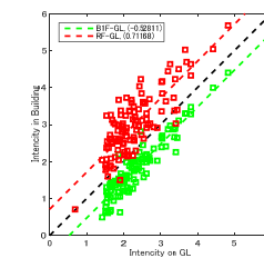
図 3.3 GLの計測震度とBIF及びRFの計測震度の関係
