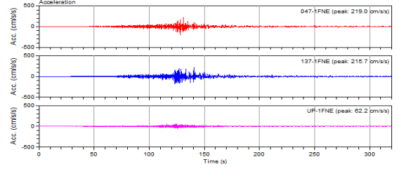
図 7.2 1 階 (O1F) の加速度記録
