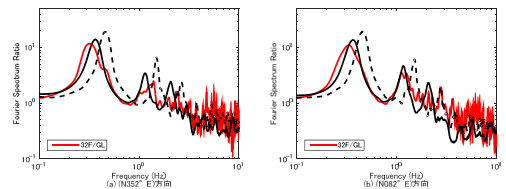
図 6.9 311地震と震度2の地震の比較(32F/G1) ※実線: 本震後、破線: 本震前
