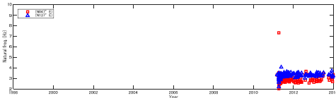
図 5.2 固有振動数 (SF/GL) の経年推移
