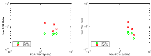
図 4.1 等価卓越振動数 (fA) と最大加速度比 (20F/GL, 1F/GL) の関係
