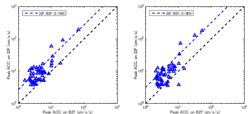
図 3.7 B2F の最大加速度と 32F の最大加速度の関係
