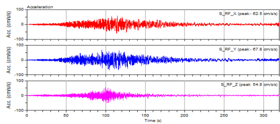
図 7.3 R階(RF)の加速度記録
