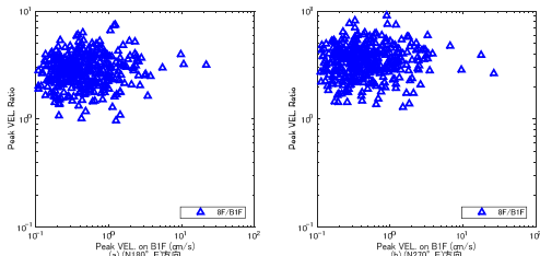
図 3.11 BIF の最大速度と 8F/BIF の最大速度比の関係
