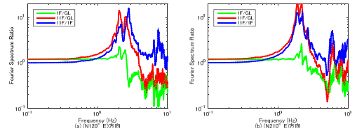
図 6.3 震度 2 の記録の平均スペクトル比(311前)
