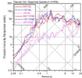
図 7.4 地表 (GL) と 1 階 (O1F) の記録の擬似速度応答スペクトル (h=5%)
