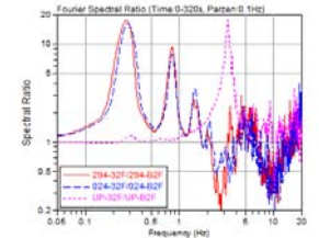
図 7.7 32 階 (32F) の B1 階 (B2F) に対するフーリエ振幅スペクトル比
