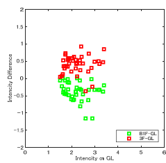
図 3.6 GLの最大震度とBIF-GL及び3F-GLの計測震度差の関係
