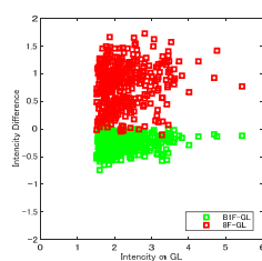
図 3.6 GL の最大震度と B1F/GL 及び 8F/GL の計測震度差の関係
