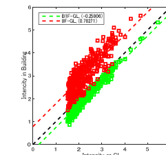
図 3.3 GL の計測震度と B1F 及び 8F の計測震度の関係
