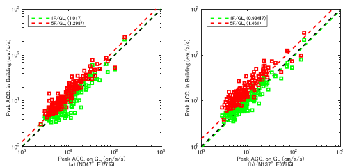
図 3.1 GL の最大加速度と 1F 及び 5F の最大加速度の関係
