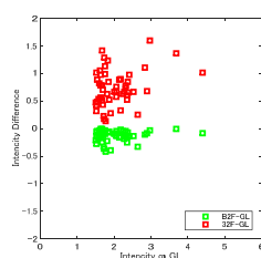
図 3.6 GL の最大震度と B2F/GL 及び 32F/GL の計測震度差の関係
