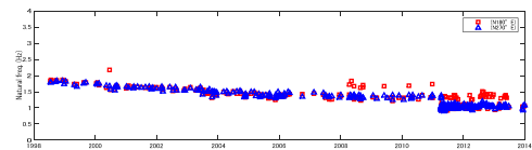
図 5.1 固有振動数 (8F/B1F) の経年推移
