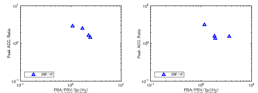
図 4.3 等価卓越振動数 (fA) と最大加速度比 (20F/1F) の関係
