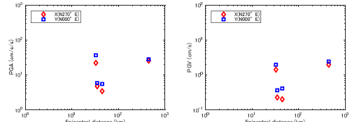
図 2.3 解析対象地震の震央距離と地表の最大加速度 (PGA) 及び最大速度 (PGV) の関係
