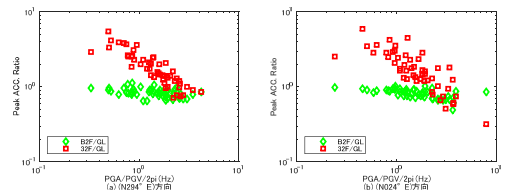
図 4.1 等価卓越振動数 (fA) と最大加速度比 (32F/GL, B2F/GL) の関係
