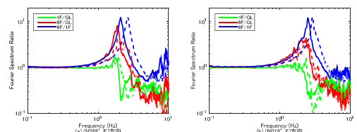
図 6.11 8.311前後の平均スペクトル比(震度4) ※実線: 本震後、破線: 本震前
