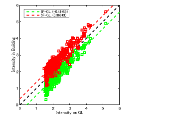
図 3.3 GL の計測震度と 1F 及び 6F の計測震度の関係
