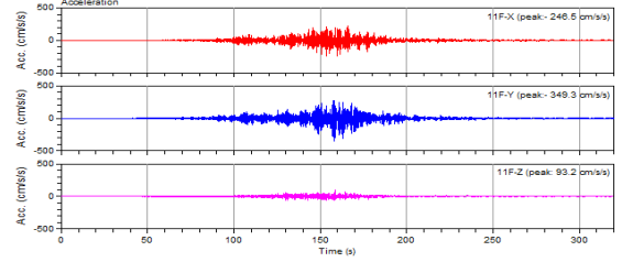
図 7.3 11階 (11F) の加速度記録
