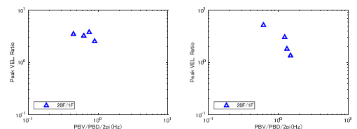
図 4.4 等価卓越振動数 (fV) と最大速度比 (20F/1F) の関係
