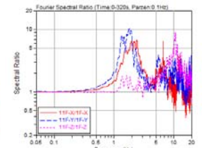
図 7.7 11階 (11F) の 1階 (O1F) に対するフーリエ振幅スペクトル比
