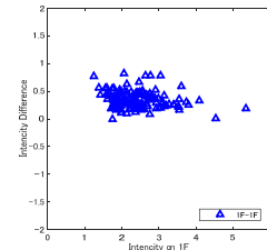
図 3.12 1F の計測震度と SF-1F の計測震度差の関係
