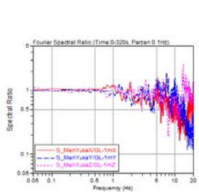
図 7.5 B1階(B1F)の地表(GL)に対するフーリエ振幅スペクトル比
