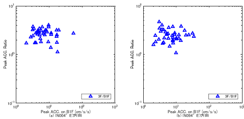
図 3.10 BIF の最大加速度と 3F/BIF の最大加速度比の関係
