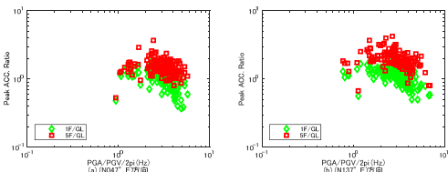
図 4.1 等価卓越振動数 (fa) と最大加速度比 (SF/GL, 1F/GL) の関係
