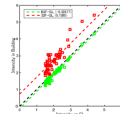
図 3.3 GL の計測震度と B2F 及び 32F の計測震度の関係
