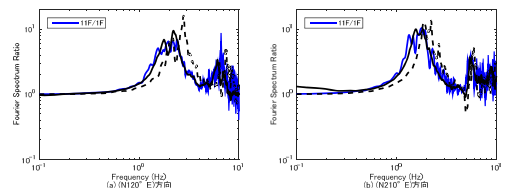
図 6.8 311 地震と震度 2 の地震の比較(1F/1F) ※実線: 本震後、破線: 本震前
