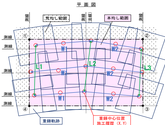
図-3.18 施工中の施工履歴データによる捨石本均しの距離計測
