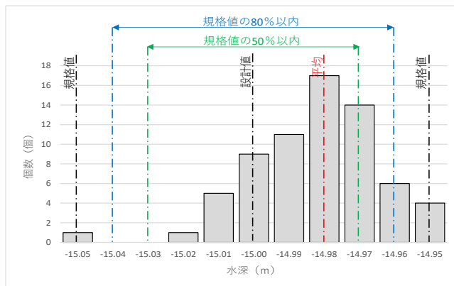
図-3.28 本均し高さの度数分布 (現地試験③より)
