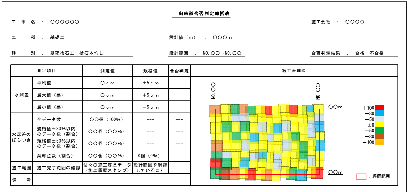
図-A.1 捨石本均し出来形管理図表作成例
