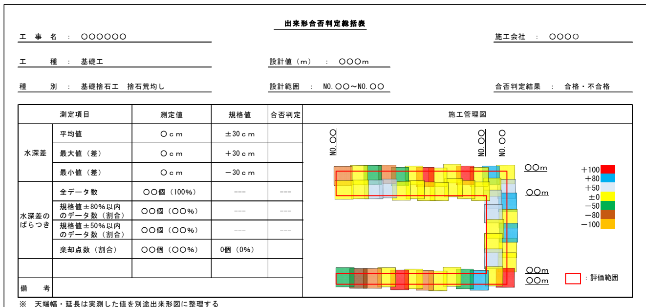
図-A.2 捨石荒均し出来形管理図表作成
