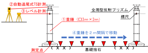
図-3.2 現地試験方法
