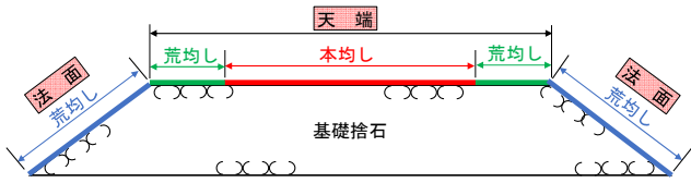
図-3.23 基礎捨石均し施工区分
