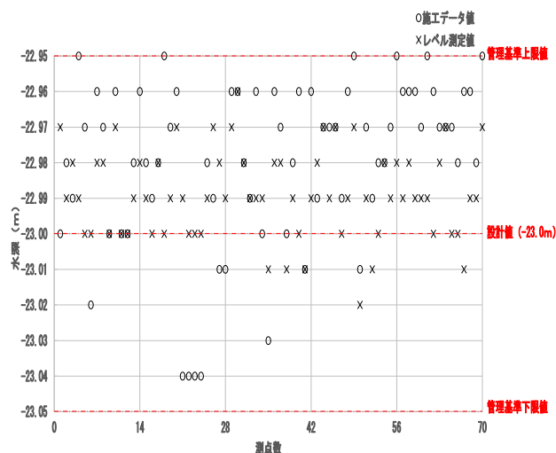
図-3.7 施工データ値とレベル測定値の比較散布図
