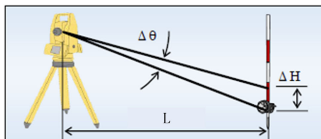
図-3.12 計測器の器械誤差 \Delta H
