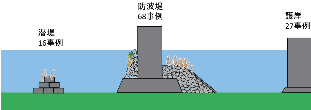
図-3.2 海藻の生育基盤の工夫が実施された構造物とそれぞれの事例数
