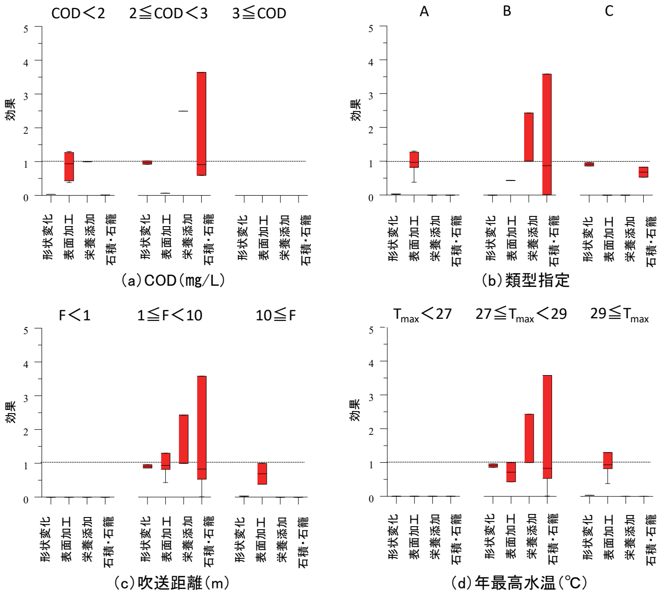
図-3.8 環境条件に対する生育基盤の工夫の効果（ホンダワラ類）
