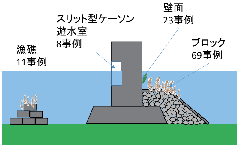
図-3.3 海藻の生育基盤の工夫が実施された箇所とそれぞれの事例数
