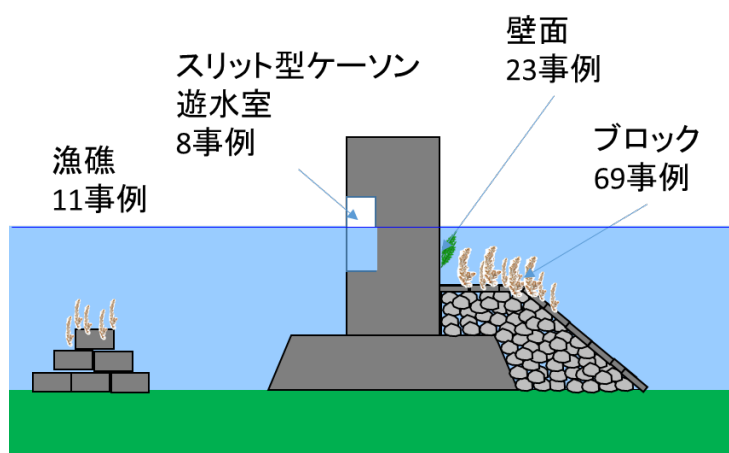
図-2 生息基盤の工夫が実施された箇所とその事例数
