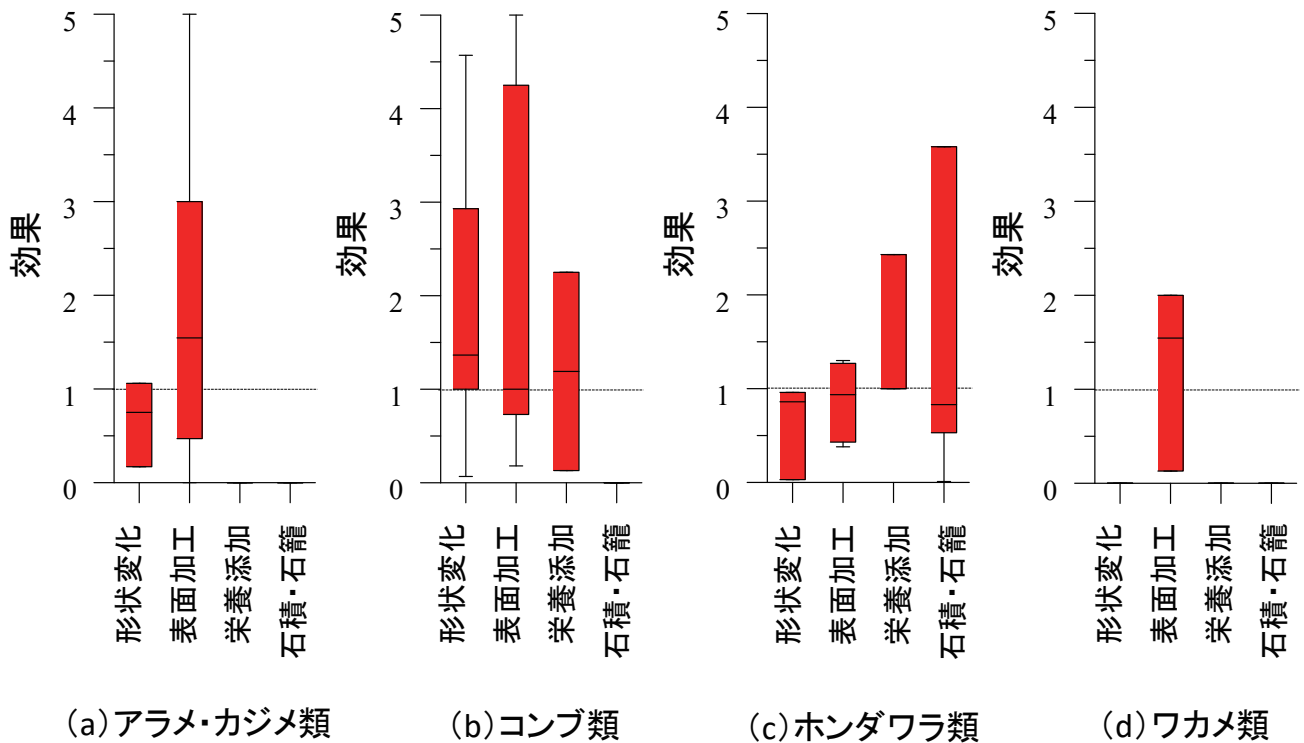
図-3.5 海藻種で区分した生育基盤の工夫の効果
