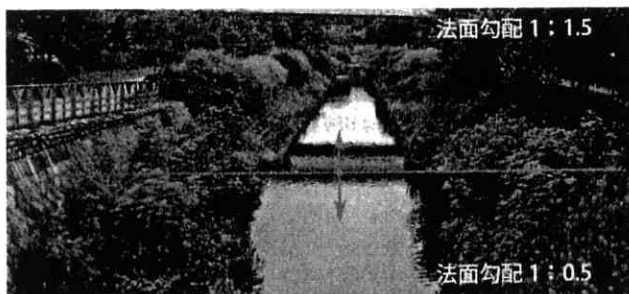
写真-5 上下流での法面勾配の違いにより、水際の植生状況が違っている例 (出典: ポイントブック)
