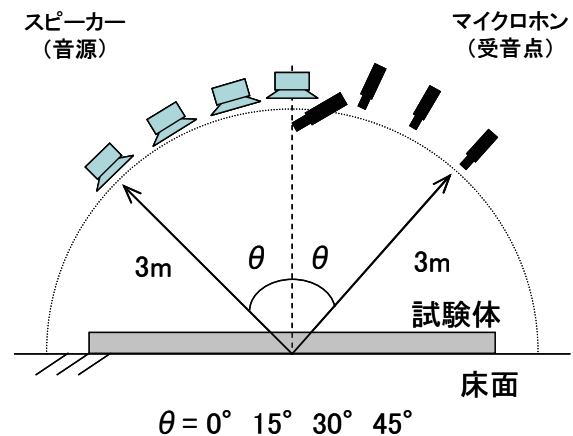
図-4 マイクロホンとスピーカの配置
