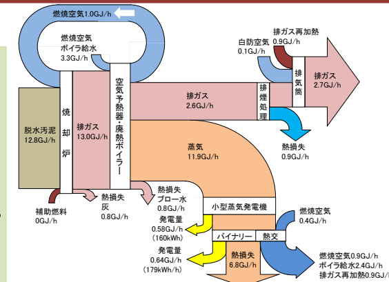
熱収支計算結果の一例(24t-DS/日)※低位発熱量基準
