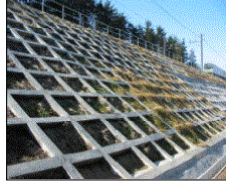
対策工(棒状補強材+のり枠工)
