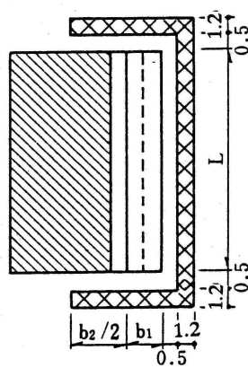
③ 平面図
