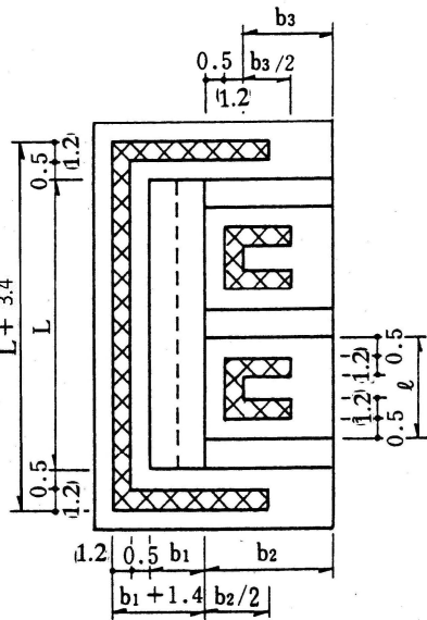
② 平面図
