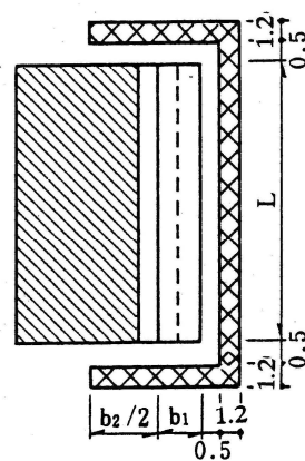
③ 平面図
