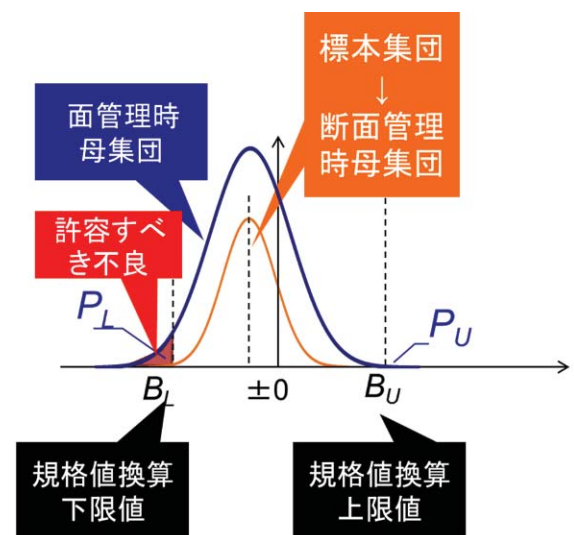
図-2 実態調査を踏まえた規格値設定
