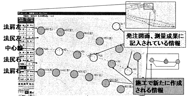
図 5 丁張りに必要な座標位置
