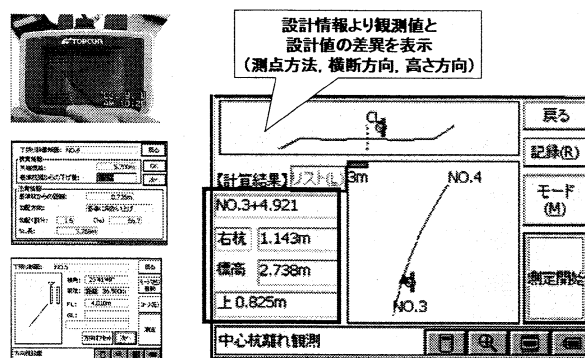
図8 データコレクタによる丁張り支援
