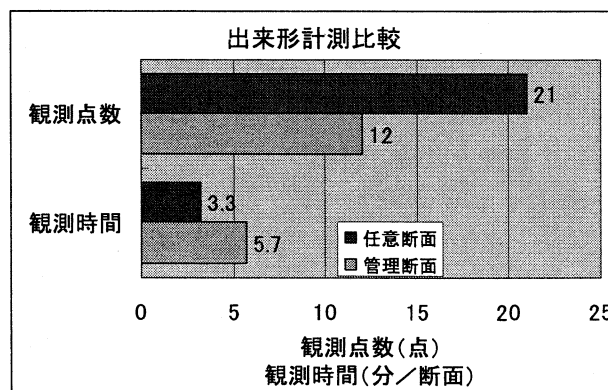
図 13 出来形計測時間
