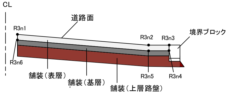
図 8 舗装の表現（例）
