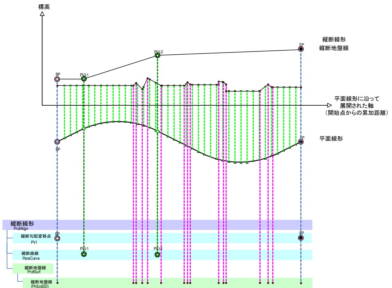
図 6 平面線形と縦断線形の対応
