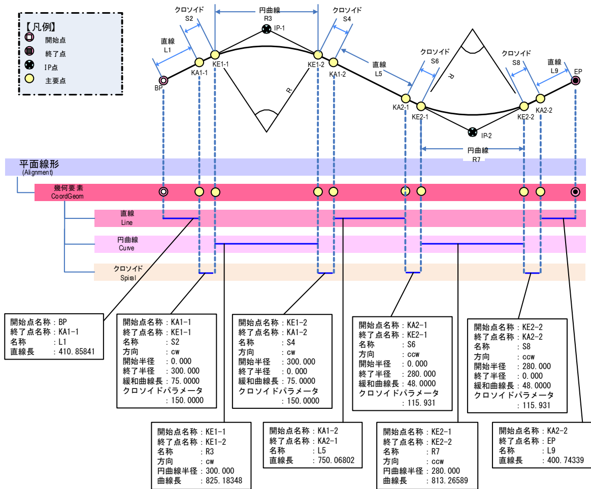
図 5 幾何要素の記述（例）
