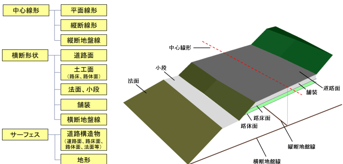
図 3 道路分野で対象とする要素とイメージ図
