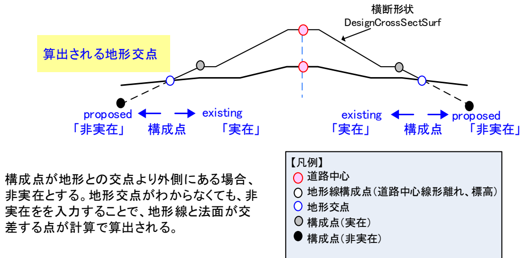
図 13 地形とのすり付けイメージ
