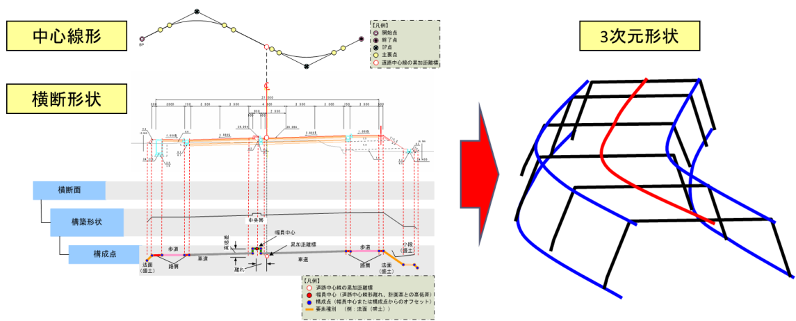
図 2 中心線形と横断形状とを組み合わせたスケルトンモデルのイメージ図
