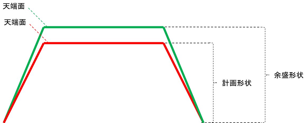
図 14 河川分野で情報化施工に必要な断面
