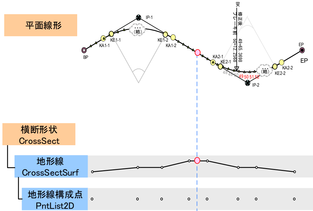
図 9 地形線の表現 (例)
