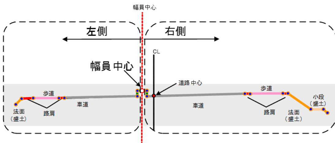
図 15 幅員中心と左右の横断構成要素イメージ
