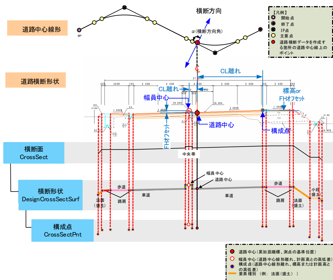
図 7 横断形状の表現（例）
