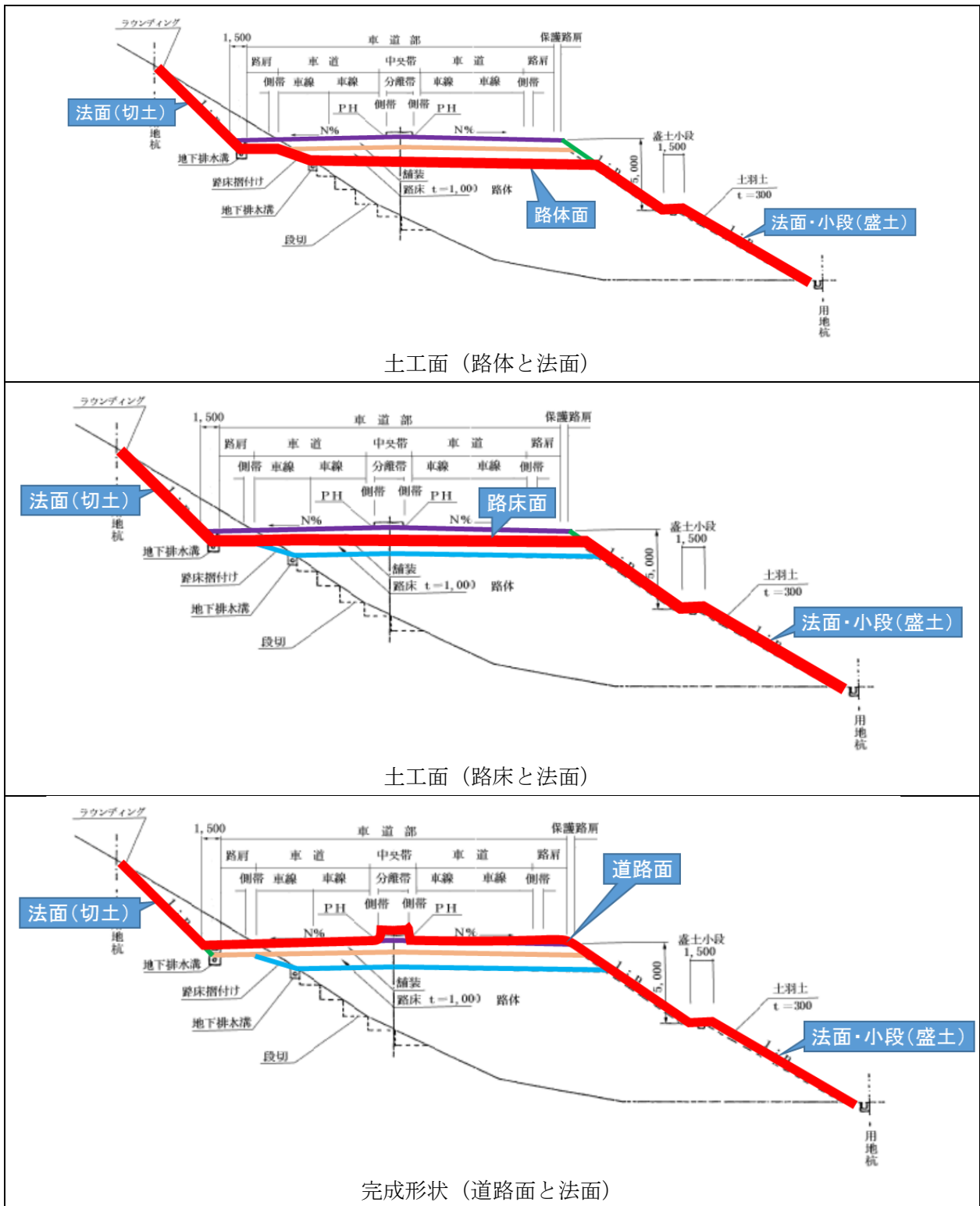
図 11 道路分野で情報化施工に必要な断面
