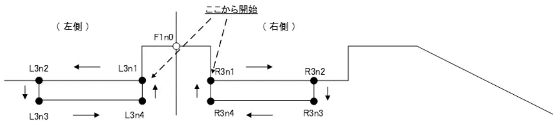
図 17 舗装などの閉じた断面の構成点を記述する順序のイメージ
