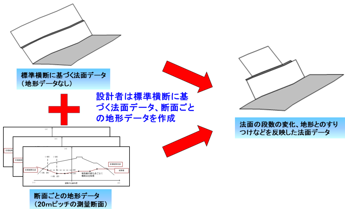
図 12 法面・地形のデータ作成
