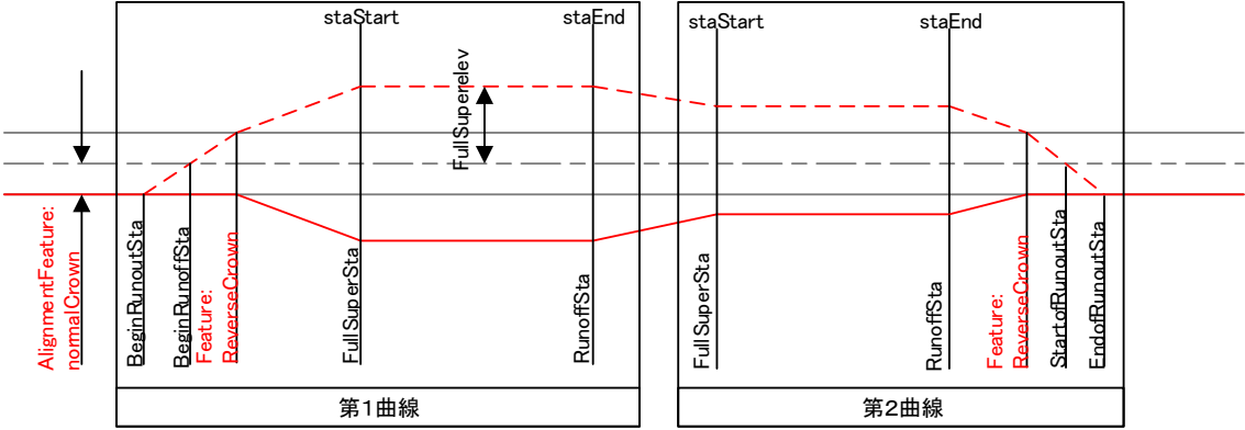
図 4-9 片勾配すりつけの例 (卵型)
